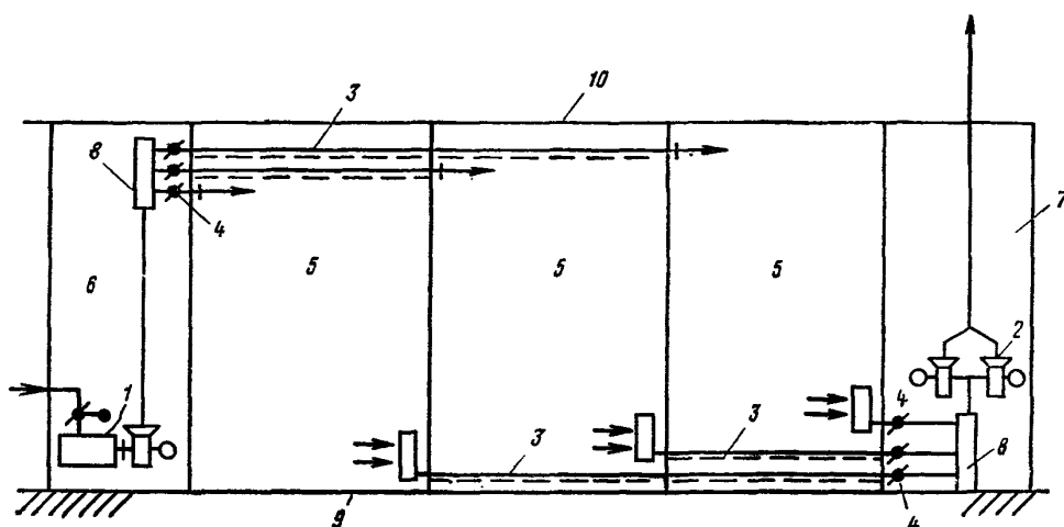
Рис. 13. Схема воздухопроводов в изолированных помещениях и складах с производствами категорий А, Б, В и Е, с выходами только наружу, расположенных в одноэтажных зданиях
