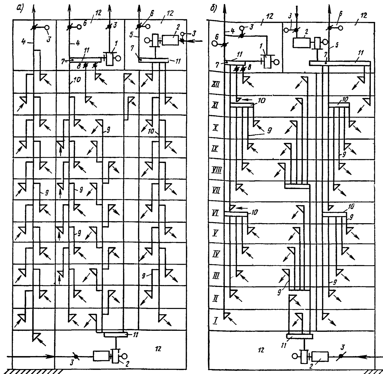
Рис. 16. Схемы воздухопроводов в многоэтажных общественных и жилых зданиях и вспомогательных зданиях предприятий
