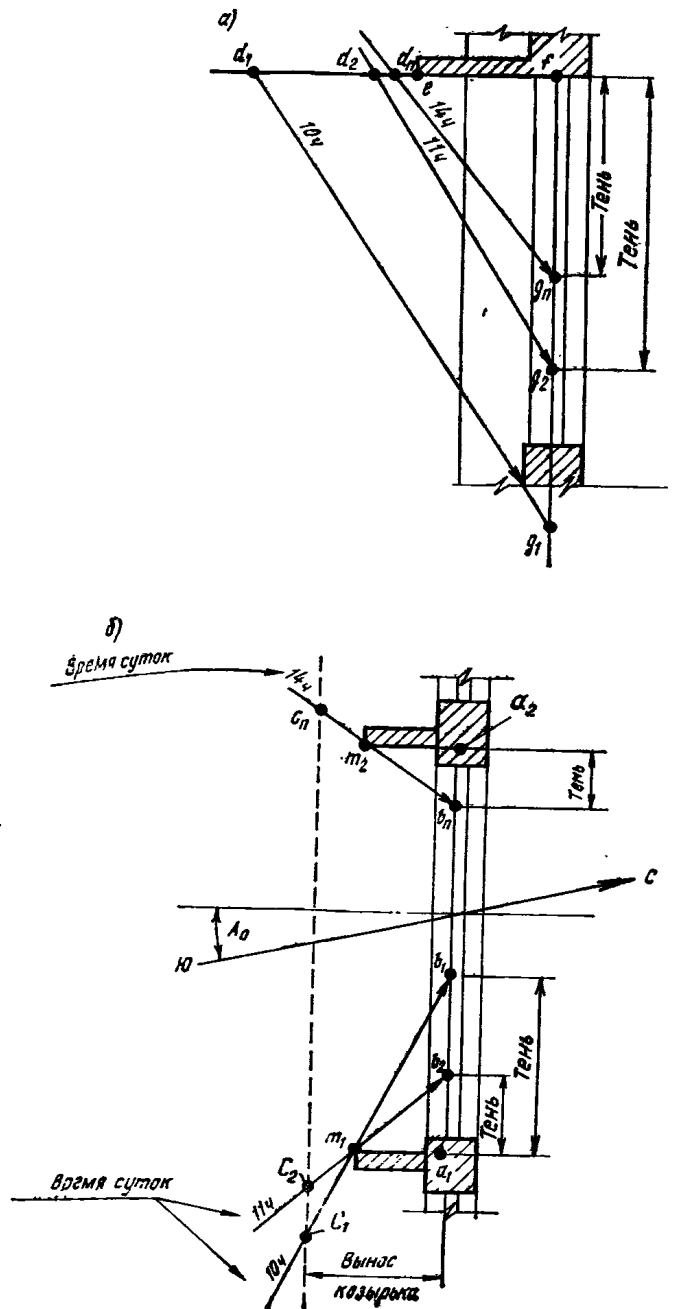
Рис. 23. Построение тени, отбрасываемой на остекление светового проема козырьком и ребрами
