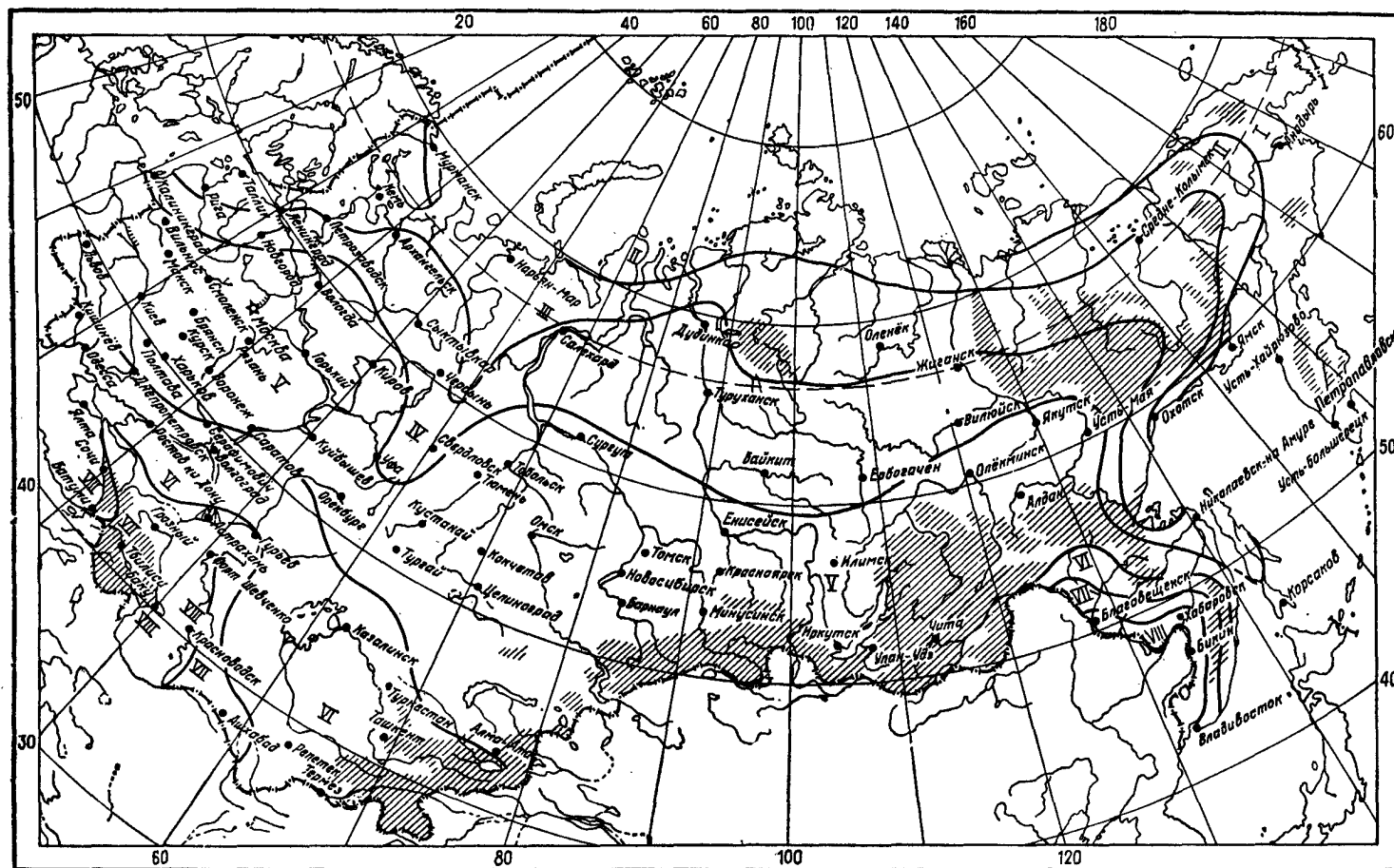
Рис. 20. Схематическая карта районирования территории СССР (районы I—VIII) по величине теплосодержания I в ккал/кг наружного воздуха в теплый период года, значения которого наблюдались 50 ч и менее в году I — I = 10,6-11,5 ; II — I = 11,6-12,5 ; III — I = 12,6-13,5 ; IV — I = 13,6-14,5 ; V — I = 14,6-15,5 ; VI — I = 15,6-16,5 ; VII — I = 16,6-17,5 ; VIII — I \geq 17,6
