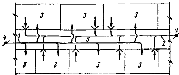
Рис. 12. Схема воздуховодов в здании коридорной системы
