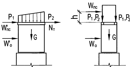
Рисунок 26.1 – Схема приложения нагрузок к перекаточной опоре.
