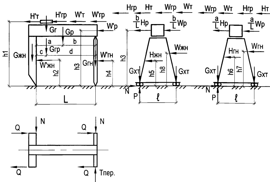
Рисунок 12.2 — Схема приложения нагрузок к козловому крану а — на жесткую ногу; б — на гибкую ногу;
