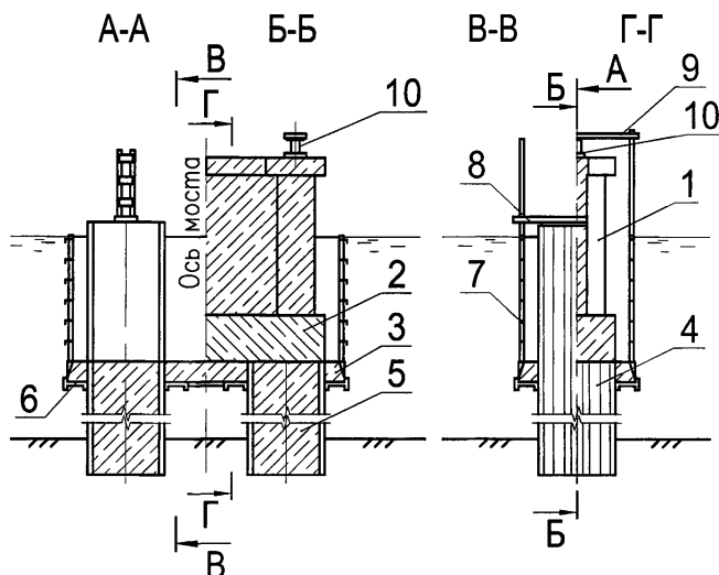
Рисунок 21.2 – Металлическое щитовое ограждение ростверка
