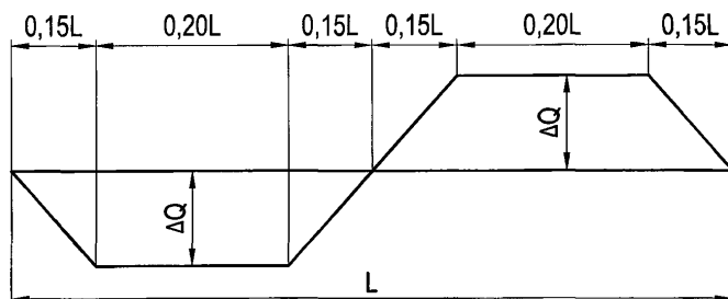
Рисунок 2 — Эпюра поперечной силы \Delta Q от волновой нагрузки
