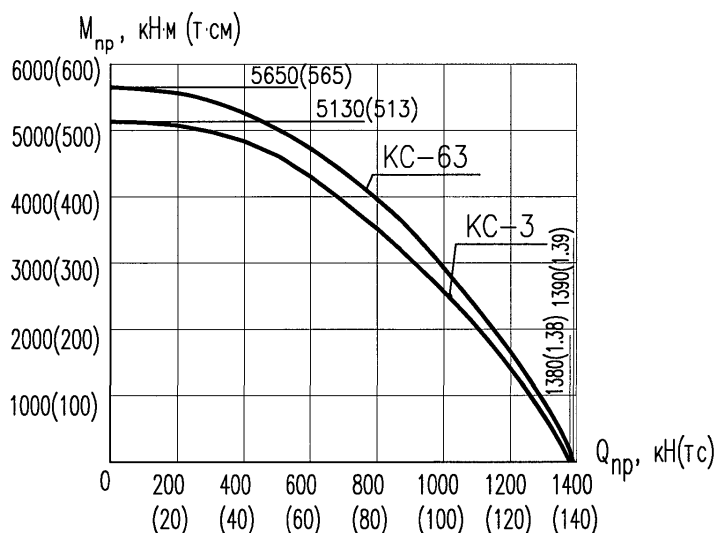
Рисунок 7.2 — График предельных усилий на понтон при изгибе в плоскости бортов и при наличии местной нагрузки (гидростатического давления) W=18 кПа ( 1,8 тс/м 2 )
