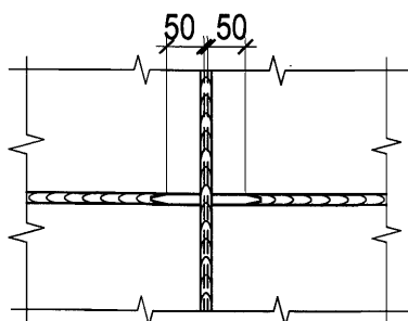
Рис. 11.3 – Пересечение стыковых швов
