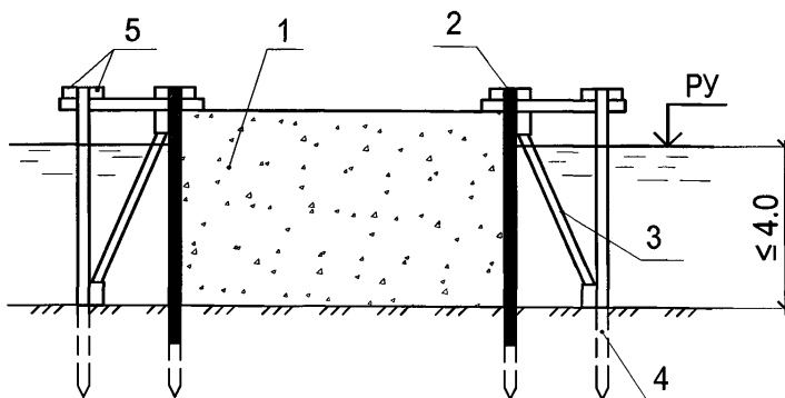
Рисунок 19.2 — Островок в деревянном шпунтовом ограждении
