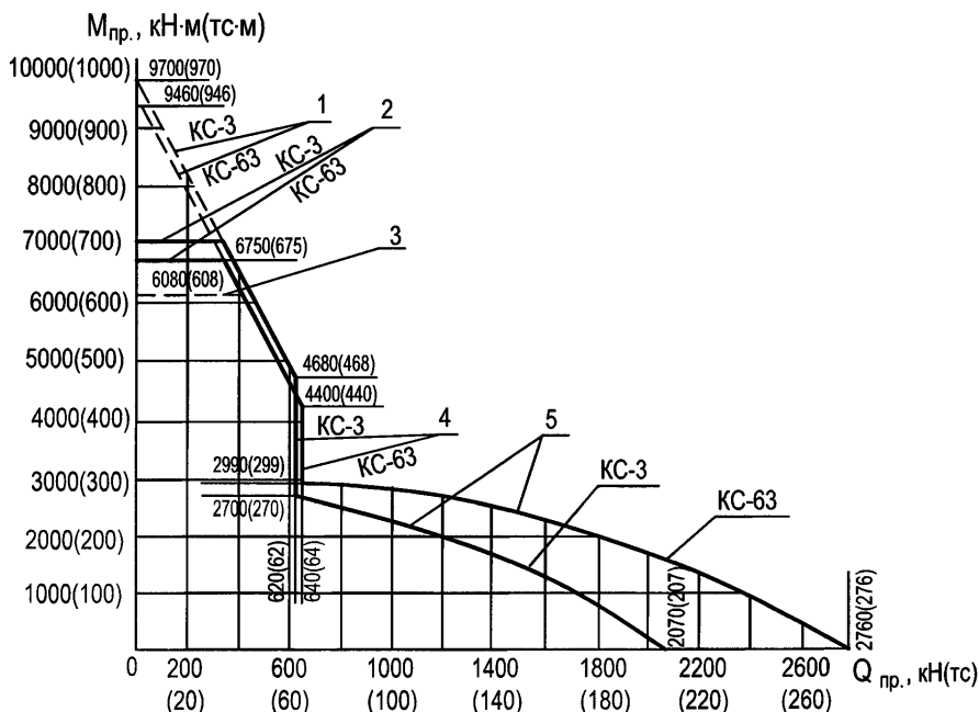
Рисунок 7.3 — График предельных усилий на понтоны КС-3 и КС-63 при изгибе в плоскости палубы.
