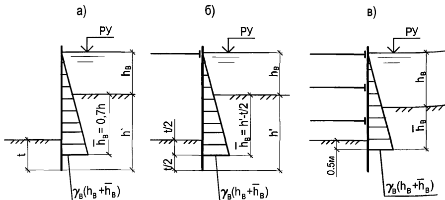
Рисунок 17.2 — Схемы для определения глубины проникания воды
