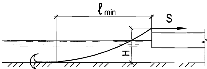
Рисунок 32.2 — Схема определения длины якорного каната.
