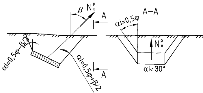
Рисунок 35.2 — Расчетная схема закопанного закладного якоря
