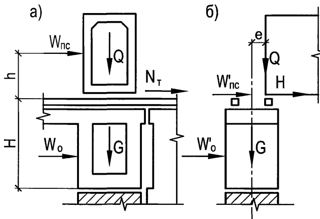
Рисунок 27.1 – Схемы приложения нагрузок к пирсам.
