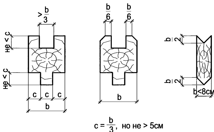
Рисунок 16.1 – Поперечное сечение деревянного шпунта
