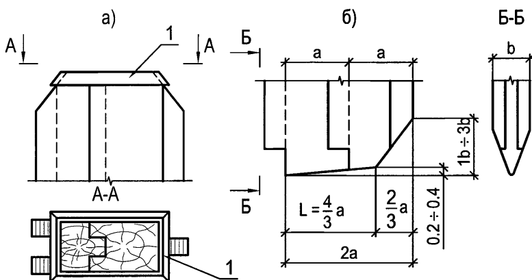
Рисунок 16.2 – Конструкция деревянных шпунтовых свай
