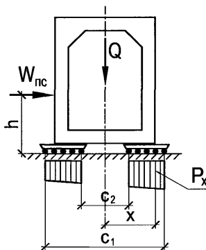
Рисунок 27.2 – Расчетная схема давления на накаточный путь.
