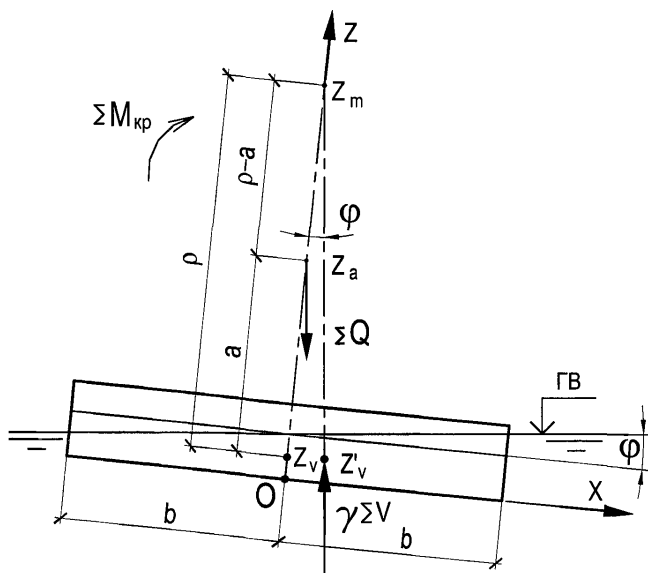
Рисунок 32.1 — Схема определения устойчивости плавучей опоры.
