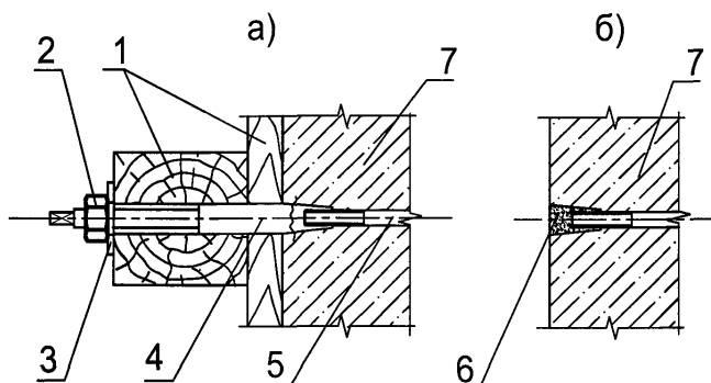
Рисунок 38.1— Тяжи со съёмными наконечниками
