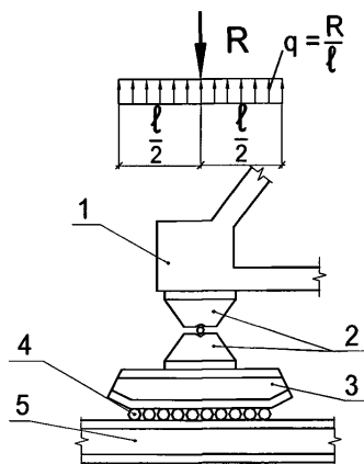
Рисунок 28.5 — Балансирное опирание узла пролетного строения на накаточные пути при продольной надвигке на плаву
