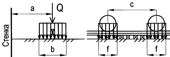
Рисунок 10.3 — К определению эквивалентной нагрузки от однорельсовой тележки на призме обрушения.
