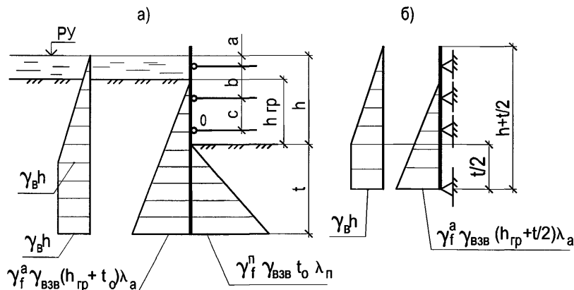
Рисунок 17.8 – Схемы расчета шпунтовых ограждений
