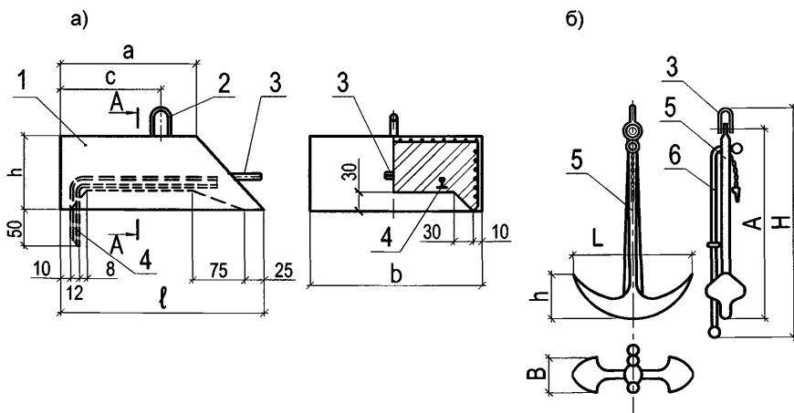
Рисунок 2 — Якоря
