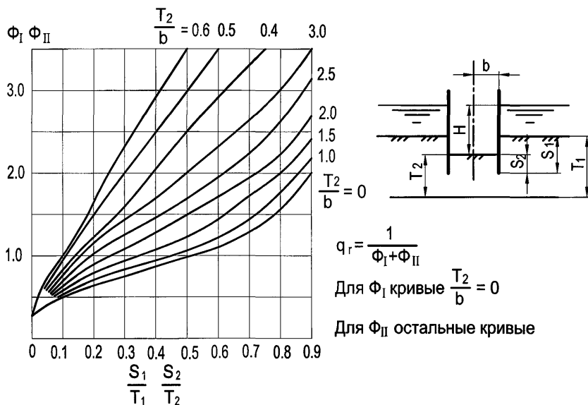
Рисунок 2 — График для определения q_r = f(S_1 : T_1 ; S_2 : T_2)
