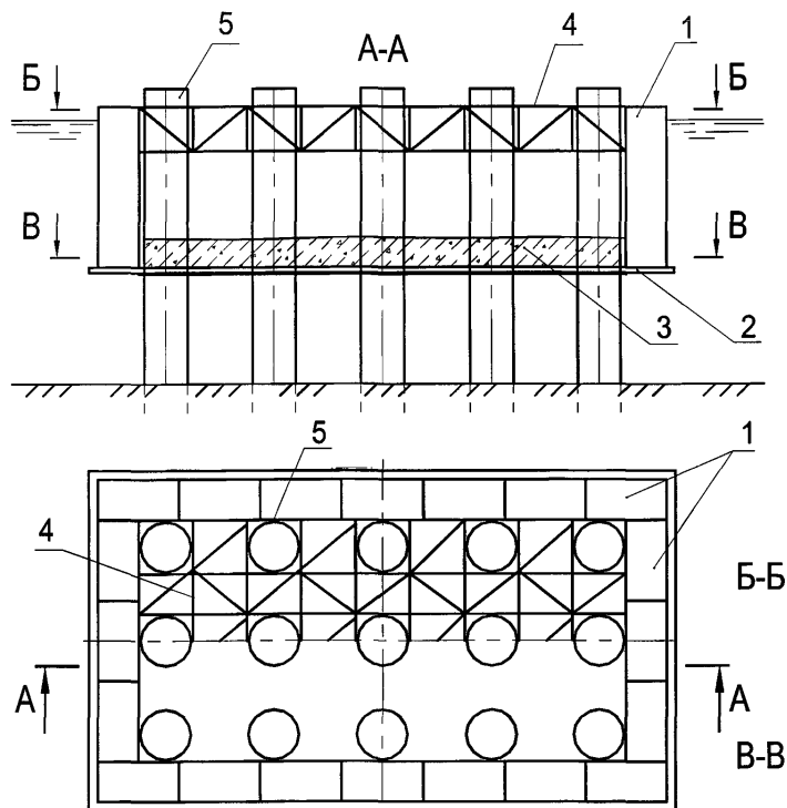
Рисунок 21.3 – Перемычка из понтонов
