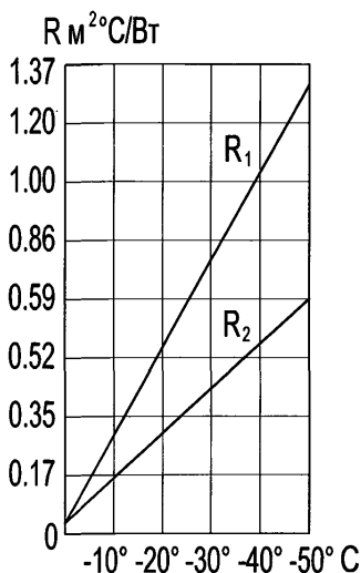
Рисунок 38.4 — Кривые зависимости оптимального термического сопротивления боковых поверхностей опоры R (в м² °С/Вт) от расчетной температуры наружного воздуха, °С ( R_1 - для торцовых поверхностей и боковых частей поверхности, прилегающих на 2 м к углам опоры; R_2 - для остальных частей боковых поверхностей).
