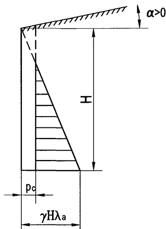
Рисунок 10.9 — К определению активного давления суглинка или глины
