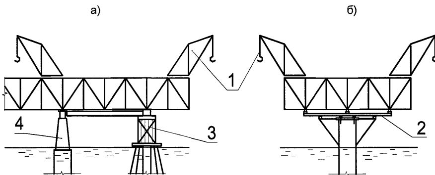
Рисунок 25.1 – Опорные устройства для уравновешенной сборки а — с опиранием на временную опору; б — закрепляемые за постоянную опору;
