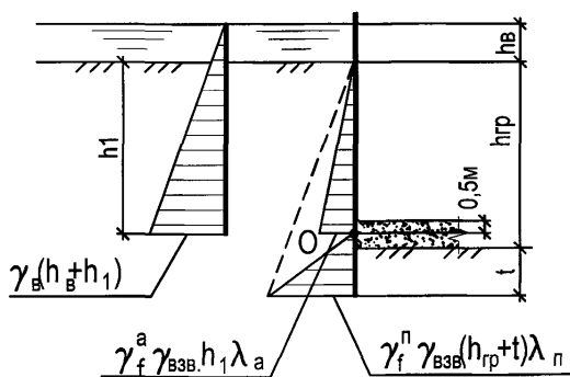
Рисунок 17.4 – Схема, используемая в расчетах шпунтовых ограждений, не имеющих распорных креплений в водонепроницаемых грунтах с применением водозащитной подушки.
