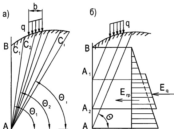
Рисунок 10.7 — К определению активного давления песка или супеси на стенку ограждений при произвольном очертании поверхности грунта и расположении на ней нагрузки
