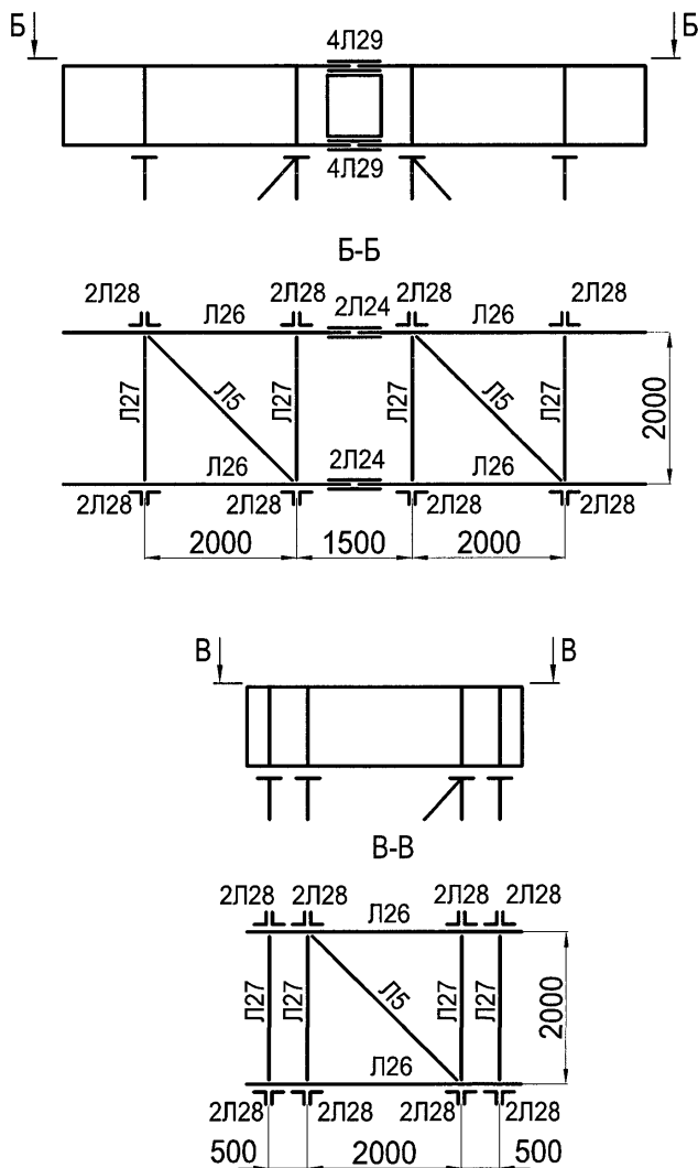
Рисунок 5.2 — Схемы компоновки сборных ростверков МИК-С2
