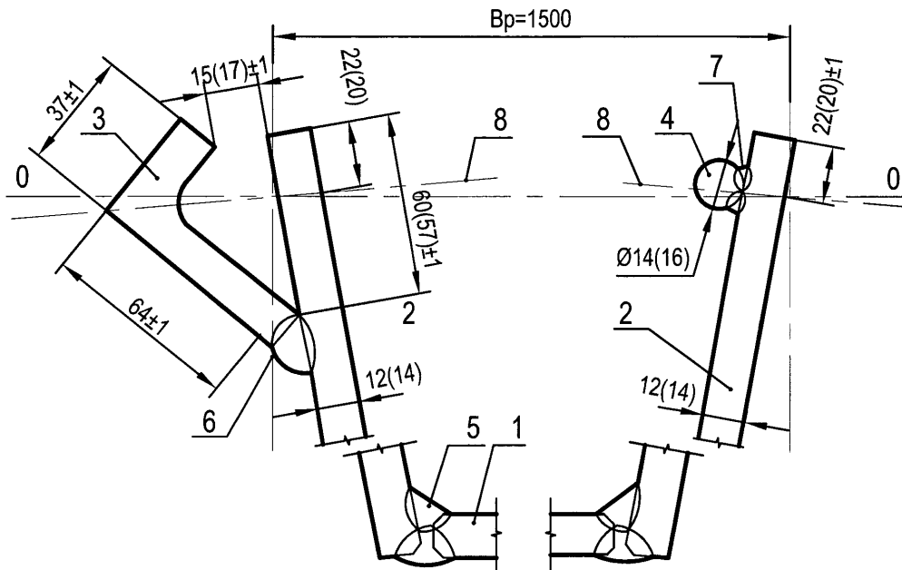
Рисунок 8.2 — Замковые элементы для панелей шириной
