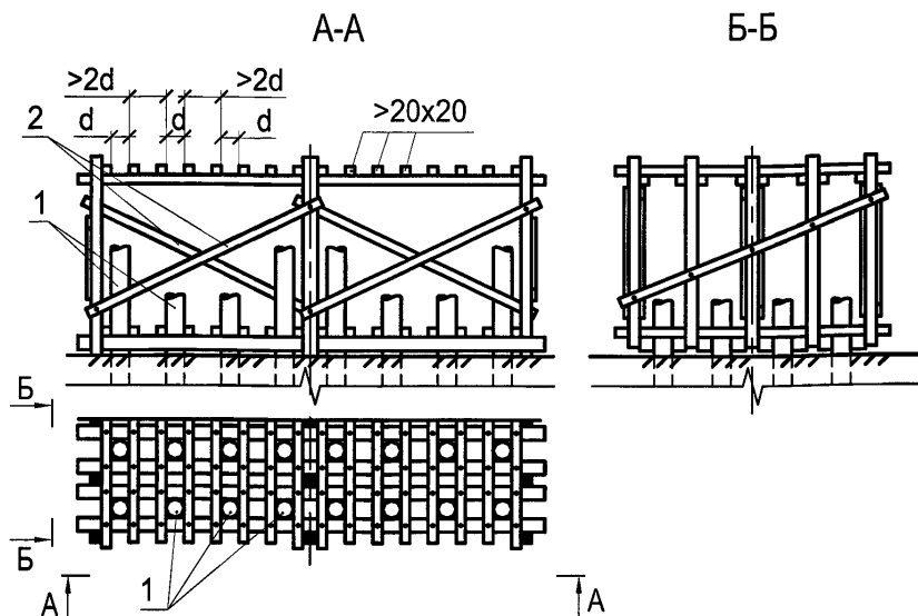
Рисунок 22.1 – Направляющий каркас из деревянных элементов
