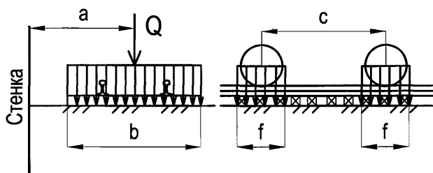
Рисунок 10.4 — К определению эквивалентной нагрузки от двухрельсовой тележки на призме обрушения.
