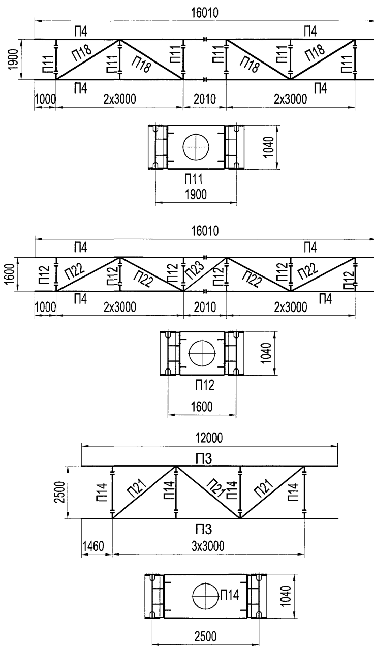
Рисунок 6.1 — Примеры монтажных схем пакетных пролетных строений МИК-П
