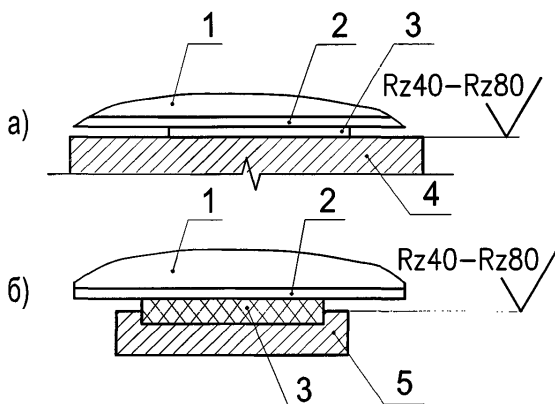
Рисунок 28.3 — Расположение в устройствах антифрикционных прокладок.
