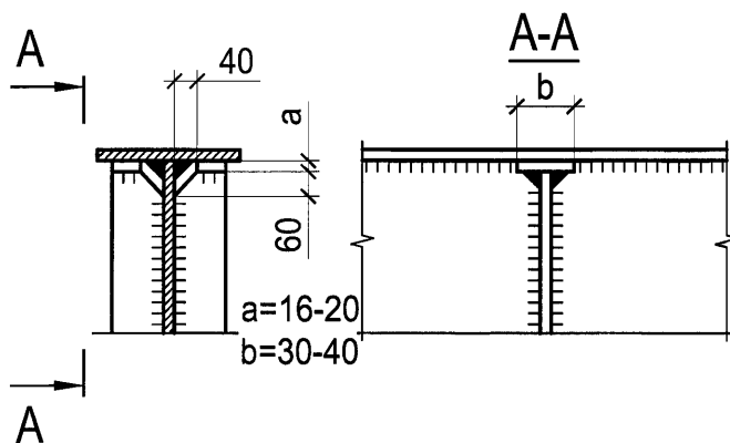
Рис. 11.1 – Примыкание ребер жесткости к поясам балки.
