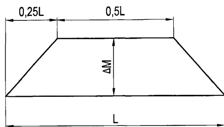
Рисунок 1 — Эпюра момента \Delta M от волновой нагрузки
