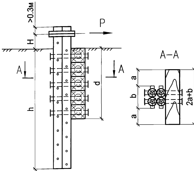
Рисунок 35.1 — Свайный якорь
