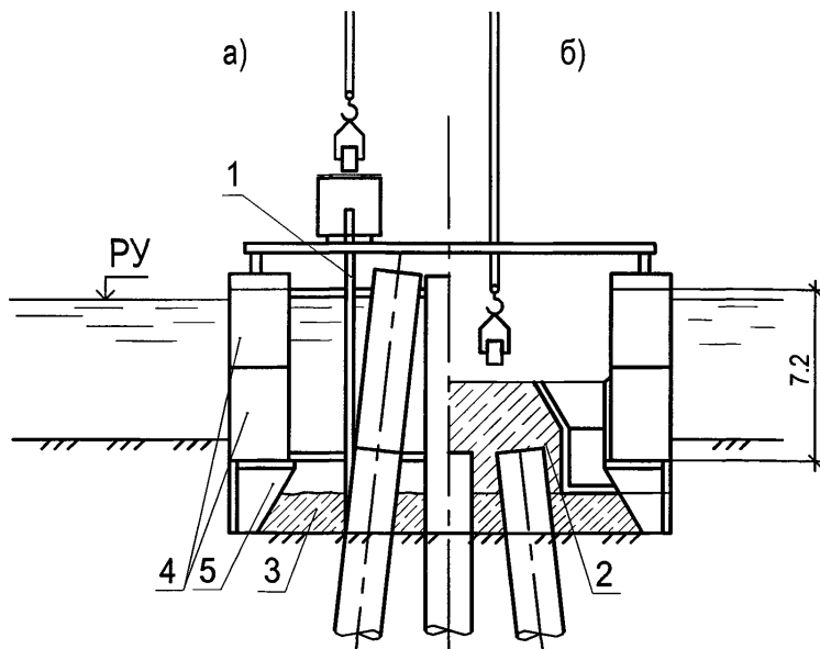
Рисунок 21.1 – Бездонный ящик из понтонов КС
