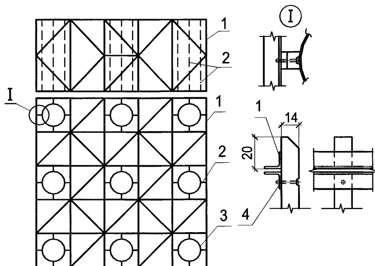
Рисунок 22.2 – Направляющий каркас из металлических элементов.
