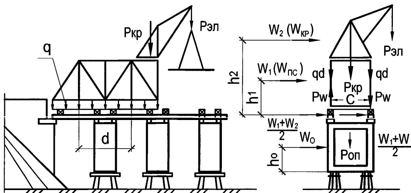
Рисунок 25.3 — Расчетная схема сборочных подмостей
