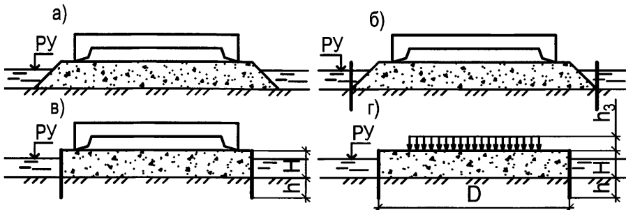
Рисунок 19.1 — Схемы искусственных островков
