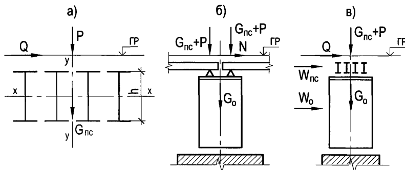
Рисунок 12.1 — Схемы приложения нагрузок в подкрановых эстакадах а — к пролетному строению; б — к опоре в продольном направлении; в — к опоре в поперечном направлении.
