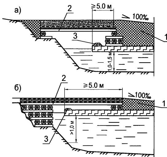
Рисунок 36.1 — Сопряжение ледовой дороги с берегом
