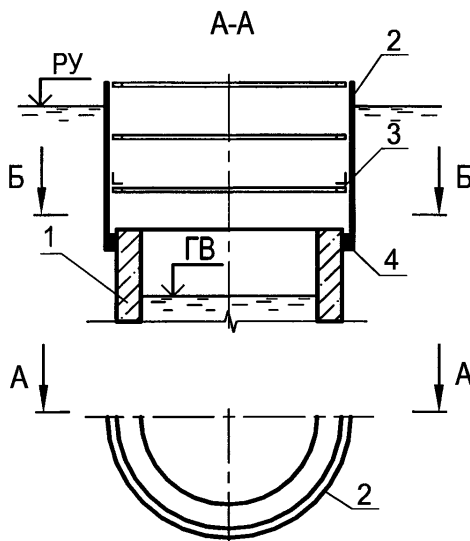
Рисунок 21.4 – Стальное ограждение верхней части круглого колодца
