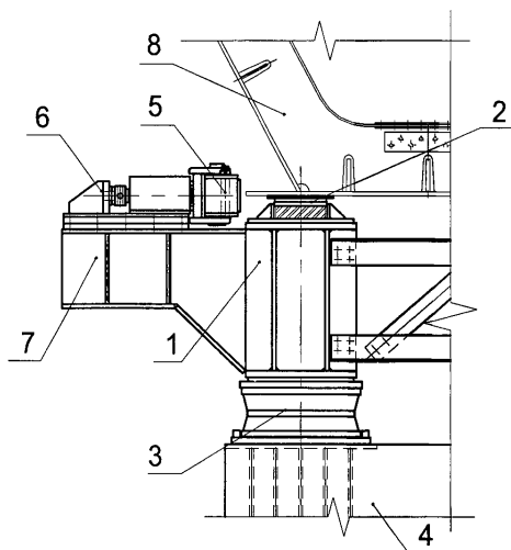
Рисунок 28.4 — Направляющее устройство
