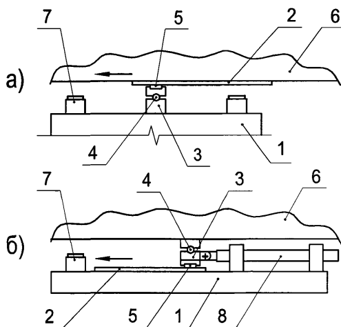
Рисунок 28.2 — Устройства скольжения циклического действия.
