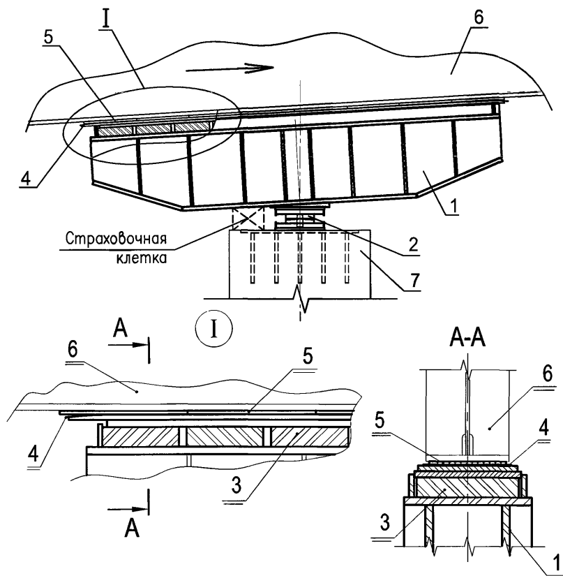
Рисунок 28.1 — Устройства скольжения непрерывного действия.
