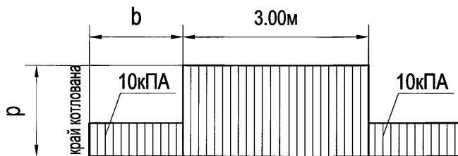
Рисунок 10.1 — Вертикальная нагрузка на призме обрушения от автотранспорта
