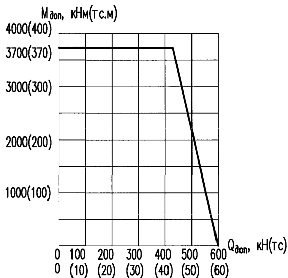
Рисунок 7.4 — График допустимых усилий на понтон УП-78
