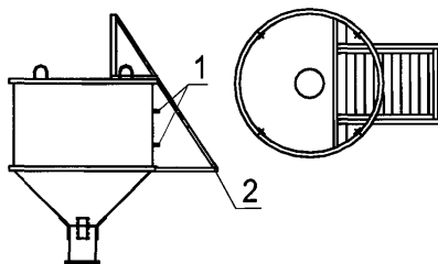
Рисунок 24.1 — Конструкция приемного бункера
