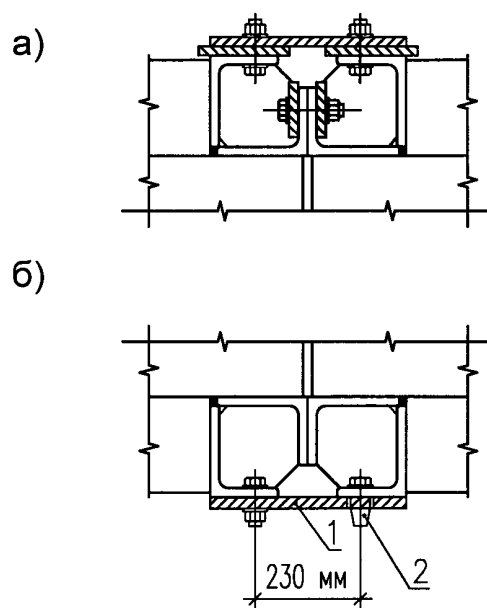
Рисунок 7.6 — Стык понтонов
