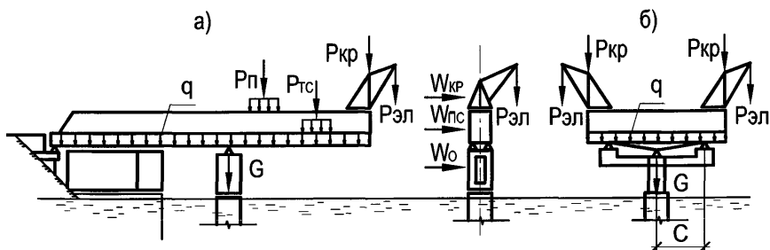
Рисунок 25.2 — Расчетные схемы нагрузок на промежуточные опоры и опорные устройства
