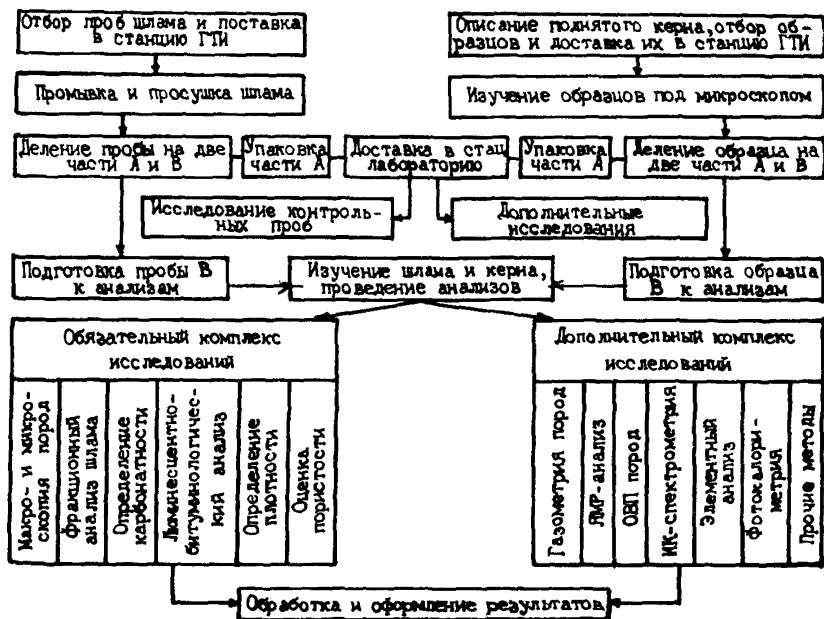
Рис. 8. Технологическая схема исследования шлама и керна.
