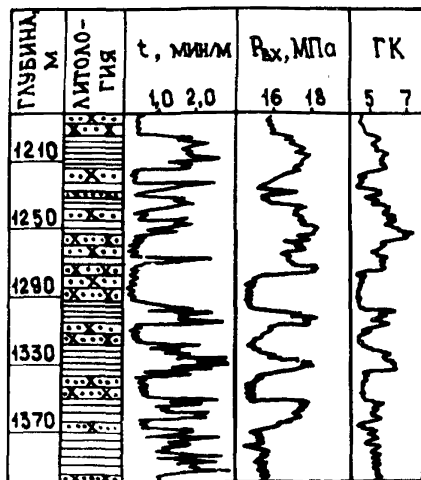
Рис. 46. Литологическое расчленение разреза (Самотлорская площадь).
