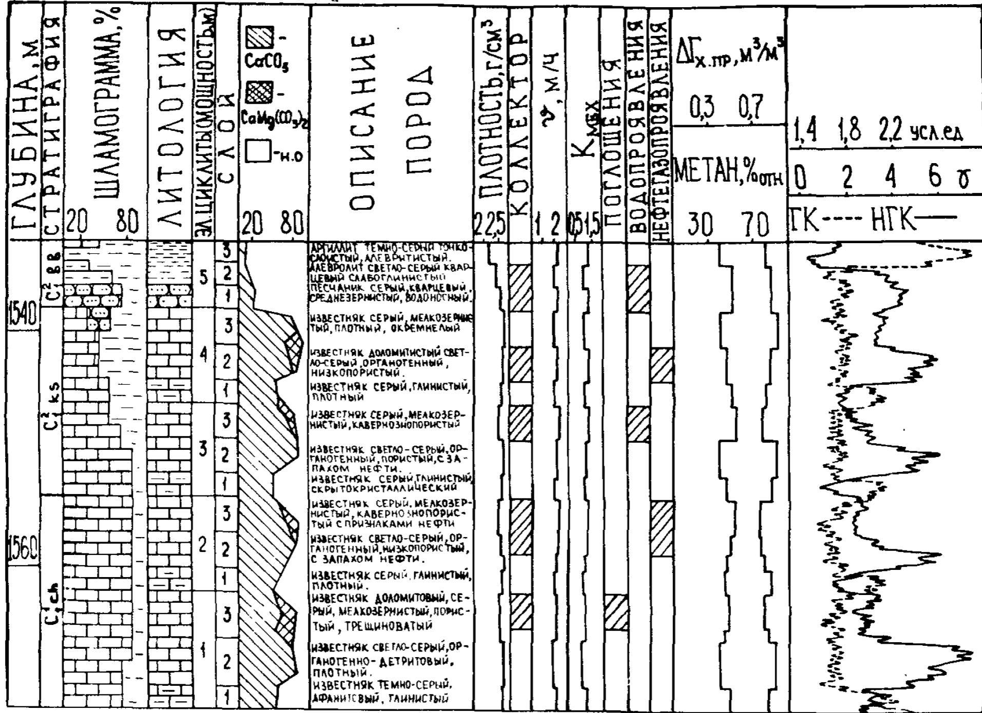
Рис. 13. Пример участка эталонно-прогнозного геологического разреза.
