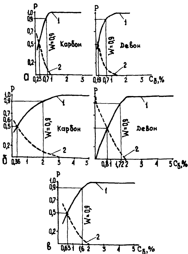
Рис. 23. Палетки вероятностного распределения C_8 в нефтеносных (1) и непродуктивных (2) отложениях нефтяных месторождений Татарии:
