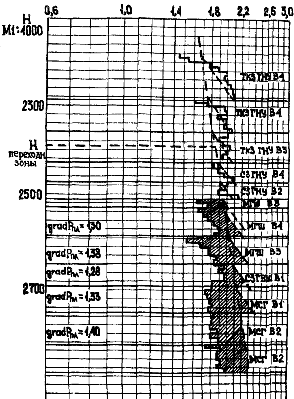
Рис. 76. Пример выделения зон АВЦД по d -экспоненте.
