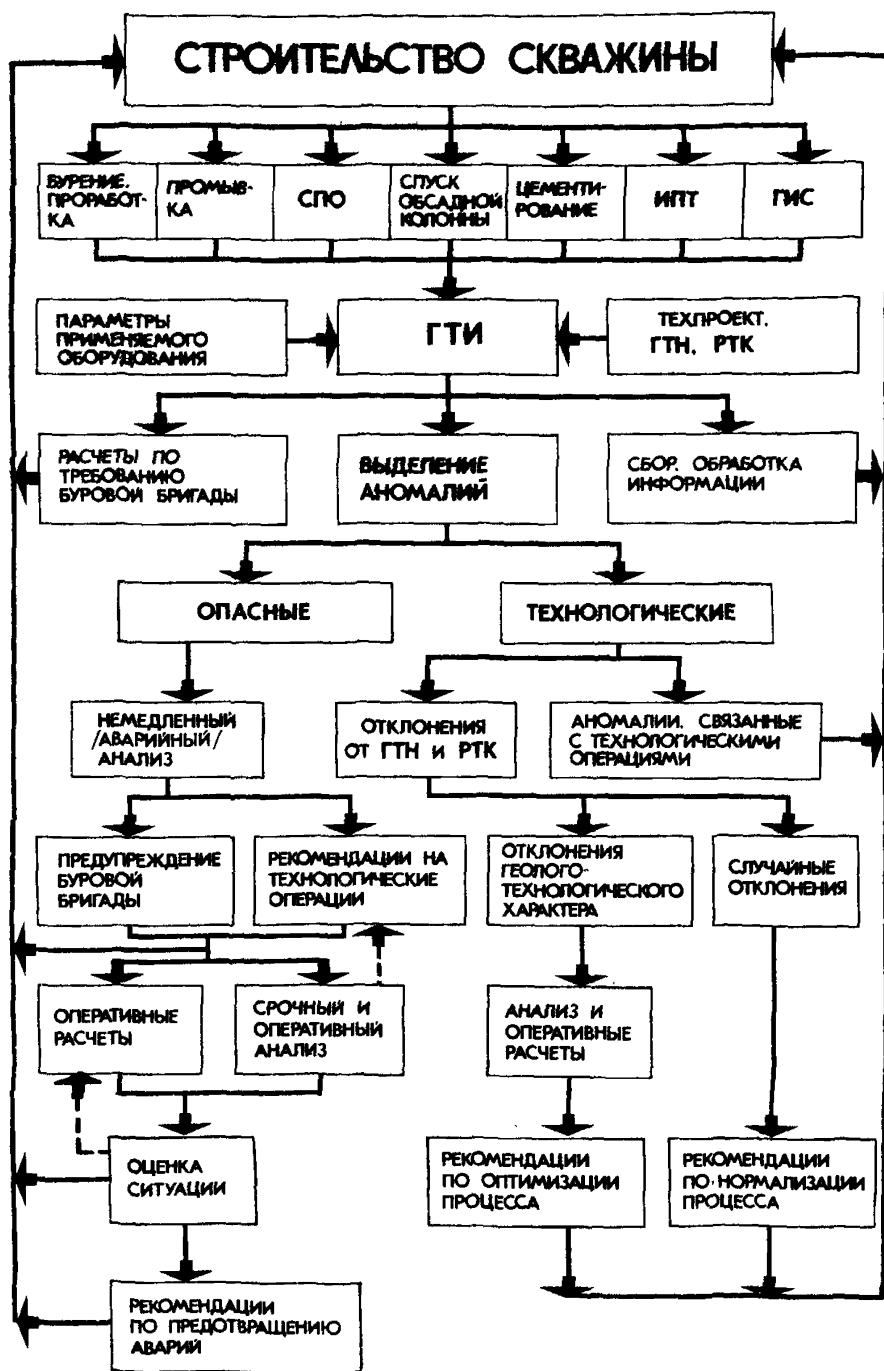
Рис. 5. Схема технологических исследований скважин.
