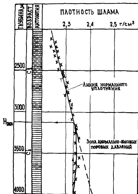
Рис. 78. Пример выделения зон АВПД по плотности шлама.
