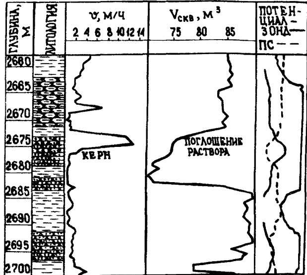
Рис. 38. Пример выделения коллектора по фильтрационному каротажу (скв. 3, пл. Пашня).
