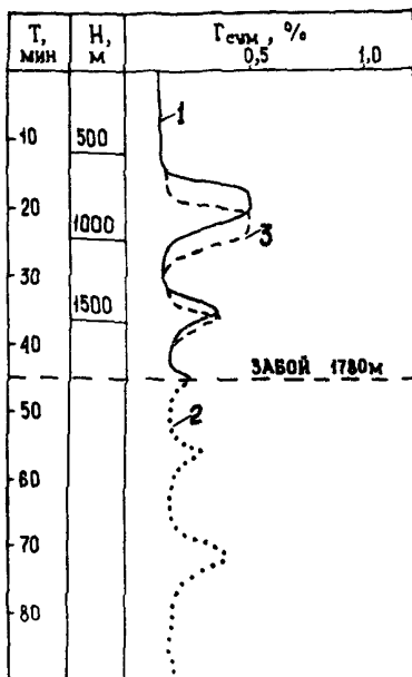
Рис. 32. Выделение нефтегазоносных пластов по результатам G_{\Sigma П} :
