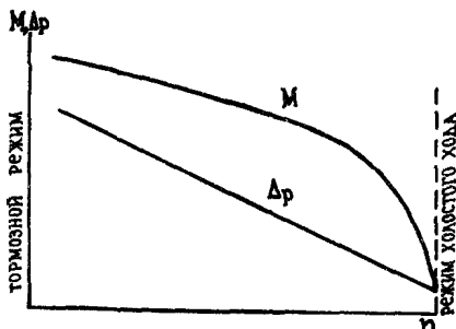
Рис. 72. Рабочая характеристика винтового забойного двигателя.
