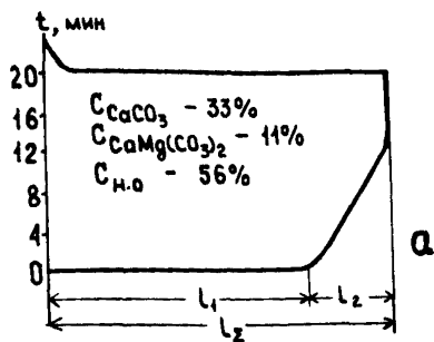
Рис. 15. Пример записи содержания кальцита и доломита в пробе шлама.
