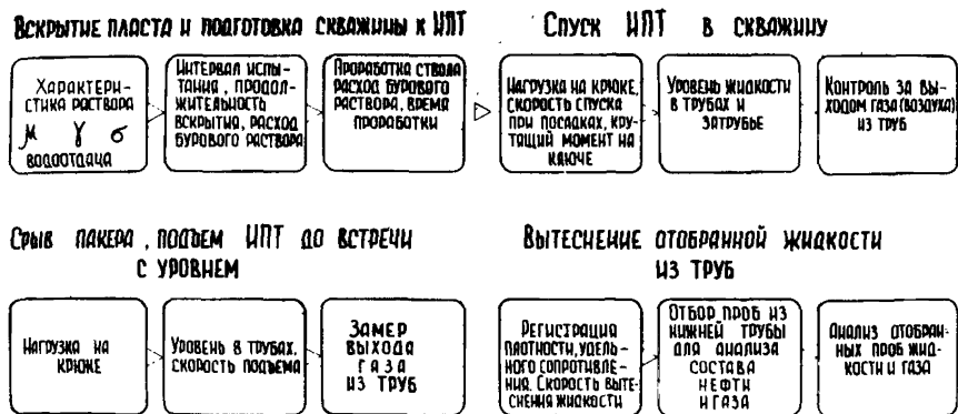
Рис. 39. Условия, определяющие качество и информативность исследуемого объекта.
