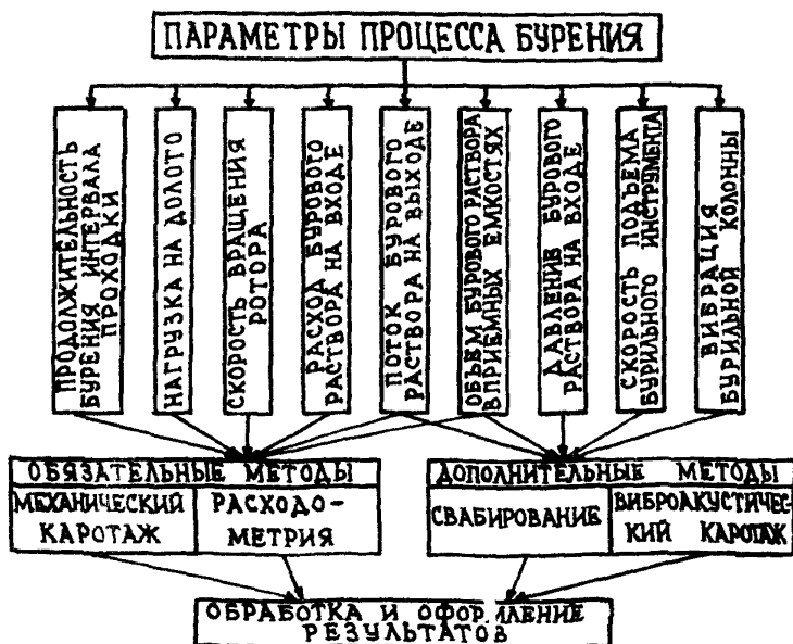
Рис. 35. Схема исследований с использованием параметров бурения.
