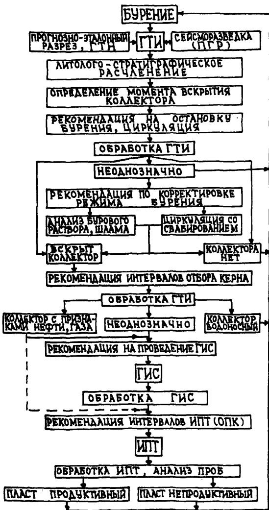
Рис. 1. Технологическая схема комплексного изучения разреза в процессе бурения.
