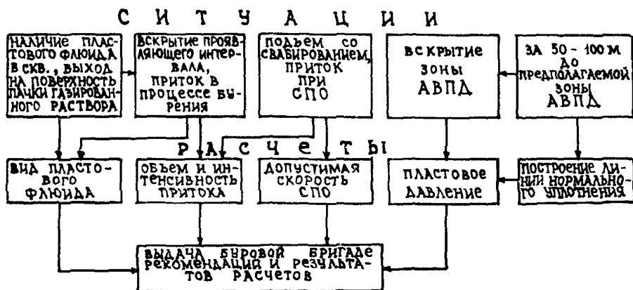
Рис. 53. Схема работ оператора по предупреждению выбросов.
