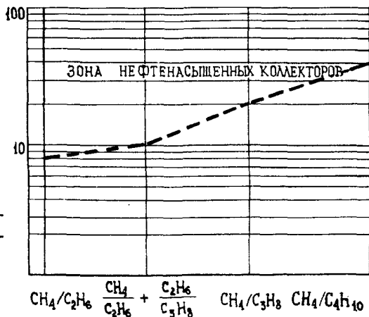
Рис. 29. Палетка флюидных коэффициентов (ГФК) для каменноугольных отложений месторождения Тенгиз (бурение на ИБР):
