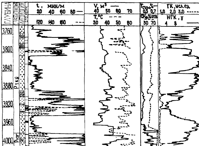
Рис. 45. Литологическое расчленение разреза по скв. 29 площади Тенгиз
