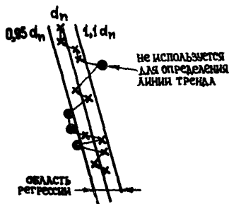
Рис. 75. Определение линии нормального уплотнения по d -экспоненте.
