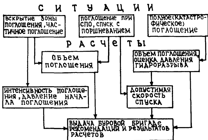
Рис. 56. Схема работ оператора по предупреждению катастрофических поглощений.
