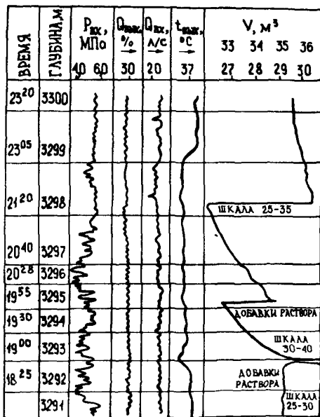
Рис. 57. Пример частичного поглощения в процессе бурения.
