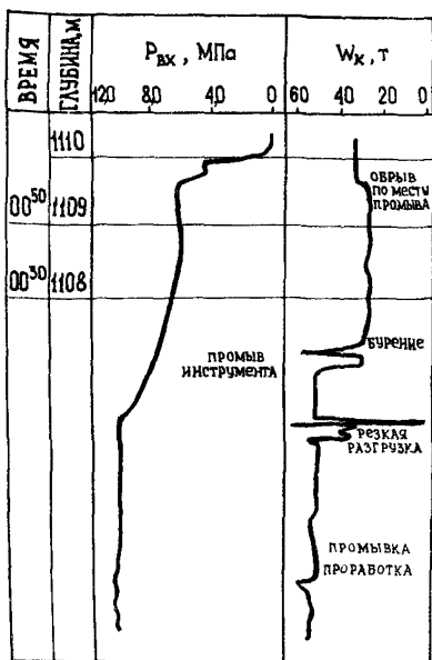
Рис. 61. Пример промыва в колонне.
