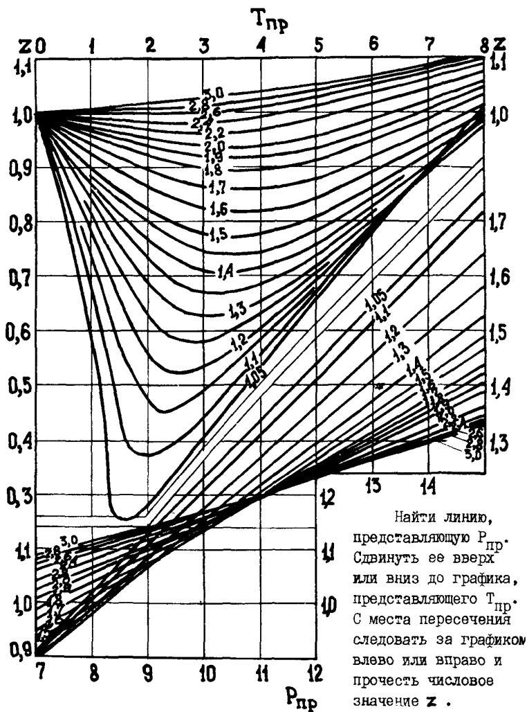
Рис. 26. Палетка для определения коэффициента сжимаемости газа z .
