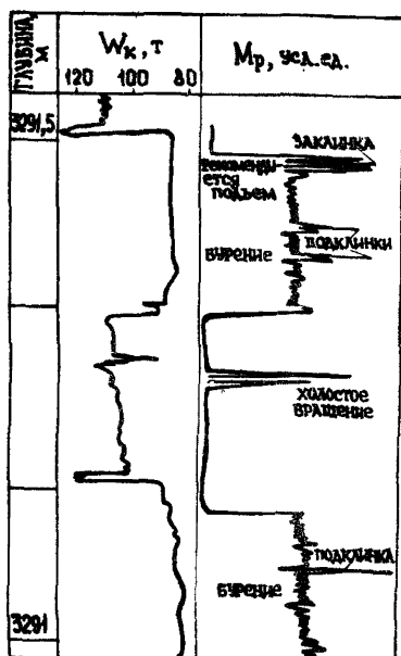
Рис. 68. Пример износа опоры долота.
