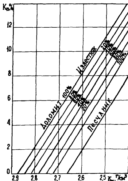
Рис. 19. Палетка для оценки пористости по плотности пород.
