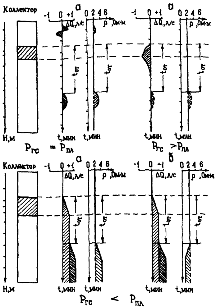
Рис. 34. Характер изменения кривых \Delta Q и \rho_{п} в зависимости от величины пластового давления и характера насыщения коллектора: а - газонасыщенный; б - водонасыщенный.
