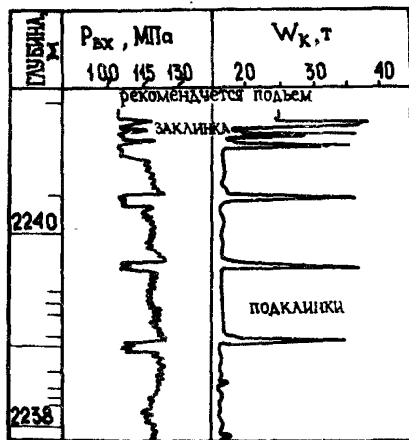
Рис. 71. Пример износа опоры долота при использовании турбобура А7ГТШ (по Э.Е.Лукьянову).
