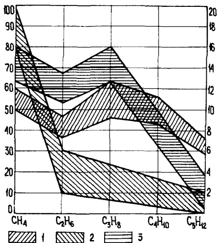
Рис. 28. Палетка раздельного анализа газа (РАГ):
