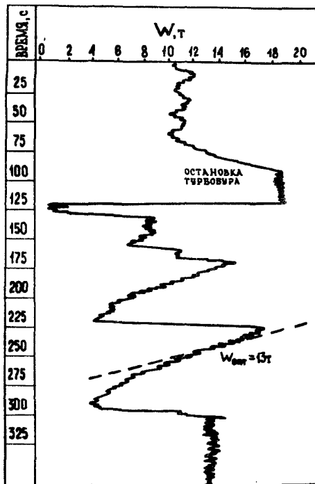
Рис. 65. Поиск оптимальной нагрузки на долото.
