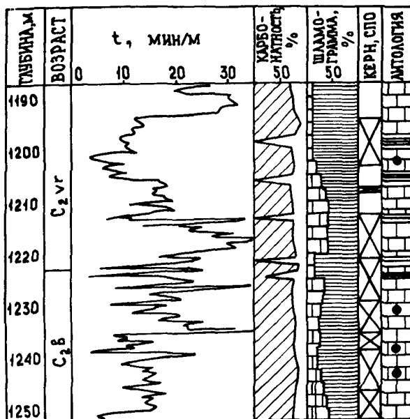
Рис. 42. Литологическое расчленение по скв. III Западно-Ножевской площади (Пермское Прикамье).
