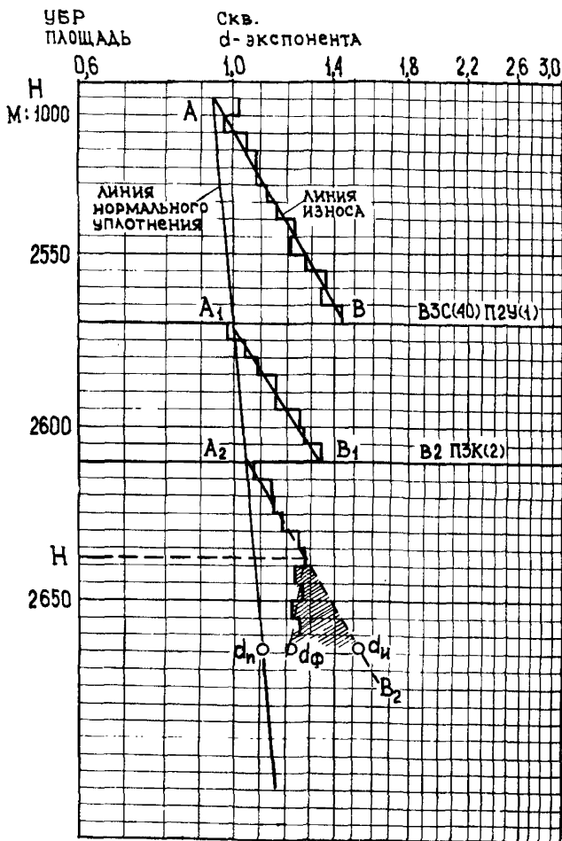
Рис. 74. График построения линии нормального уплотнения.
