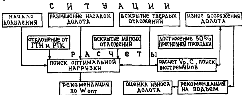
Рис. 64. Схема работ оператора по оптимальной отработке долота.
