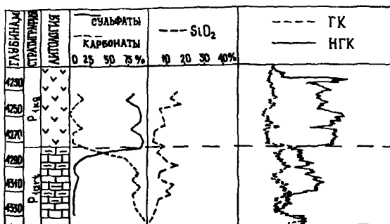
Рис. 22. Пример выделения кровли артинских отложений по результатам ИК-спектроскопии шлама (скв. 4Г, пл. Тенгиз).
