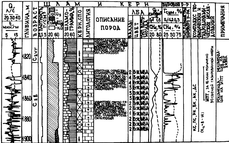
Рис. 52. Выделение продуктивных нефтеносных пластов в процессе бурения скв. 81 Уньвинской площади (Пермское Прикамье).
