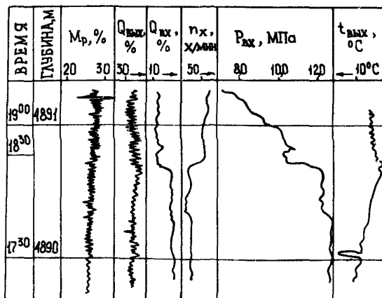
Рис. 62. Пример промыва поршня бурового насоса.
