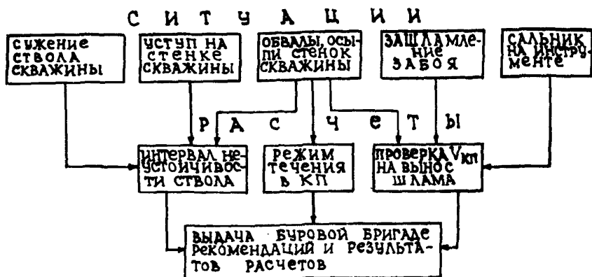
Рис. 59. Схема работ оператора по предупреждению прихватов инструмента.
