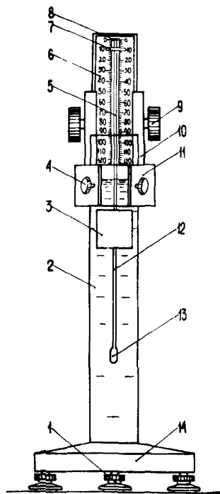
Рис. 18. Ареометрический плотномер шлама.
