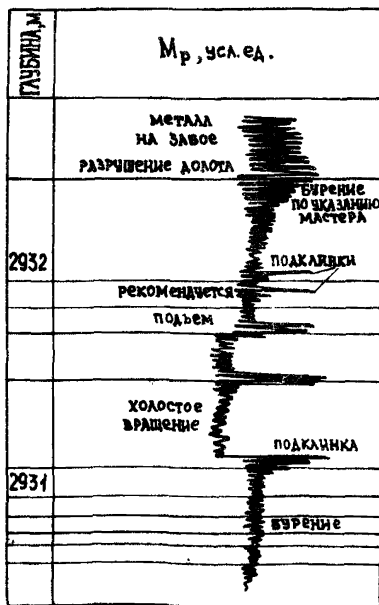
Рис. 69. Пример аварийного износа опоры долота.
