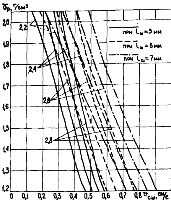
Рис. 10. Палетка для определения скорости оседания шлама.
