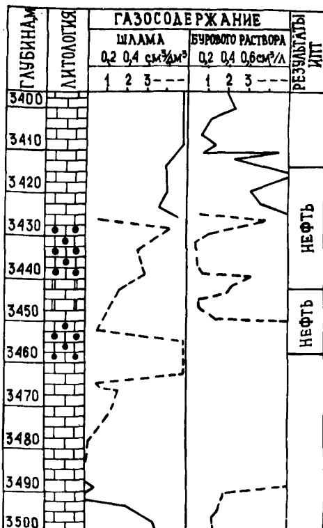
Рис. 20. Пример выделения нефтенасыщенного коллектора по газометрии шлама.
