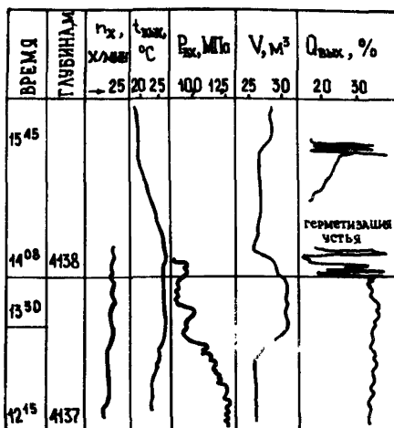
Рис. 54. Пример нефтегазопроявления в процессе бурения.
