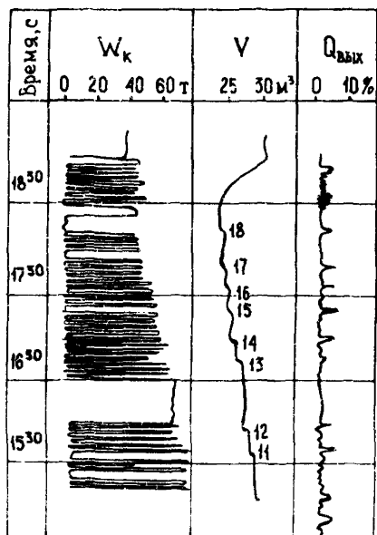
Рис. 55. Пример притока в процессе подъема инструмента.
