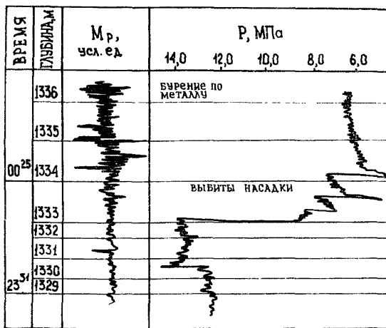
Рис. 63. Разрушение и выпадение насадок долота.
