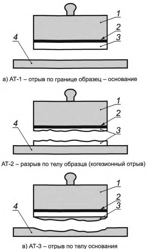
Рисунок 2 — Основные характерные виды отрыва образцов при определении прочности сцепления с основанием
