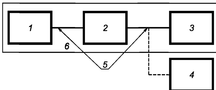
Рисунок 1 — Блок-схема установки для сличения ваттметра с РЭСМ
