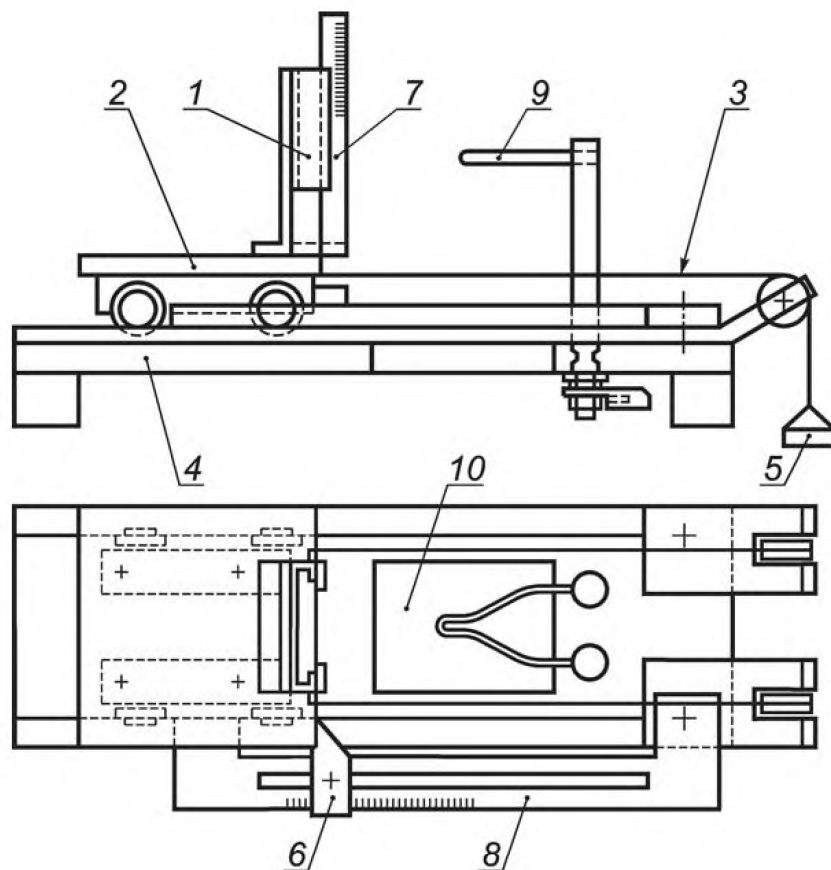
1 — опора для образца; 2 — тележка; 3 — натяжной канат; 4 — плита основания; 5 — груз; 6 — регулируемый упор; 7 — линейка для измерения пламени; 8 — линейка для измерения проникновения; 9 — раскаленная проволока (см. рисунок 8); 10 — отверстие в фундаментной плите для частиц, падающих с образца
