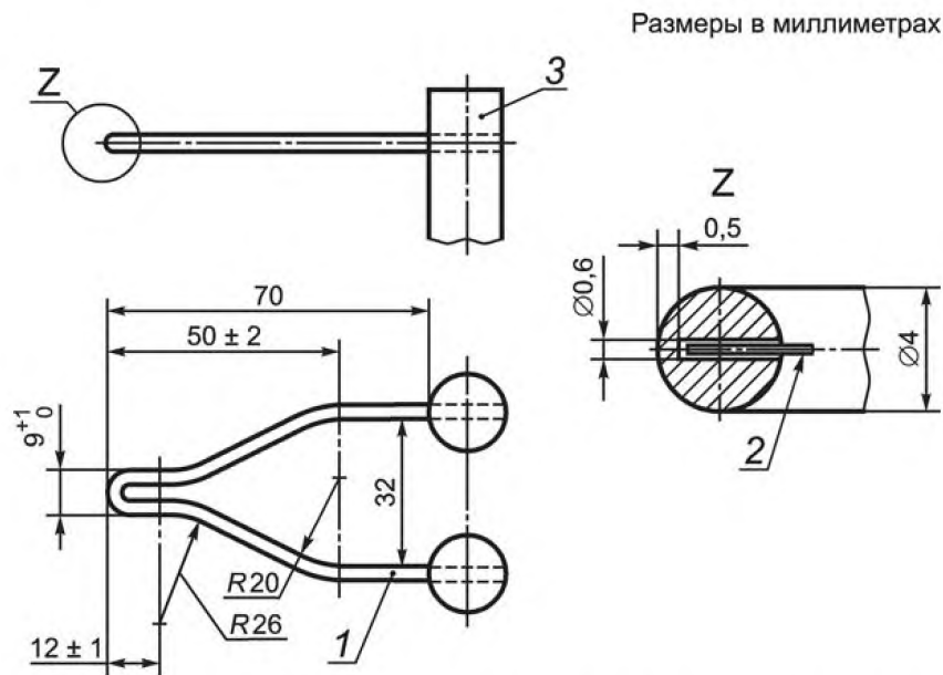
Рисунок 8 — Раскаленная проволока и положение термопары (Ранее — рисунок 7 в редакции 3)
