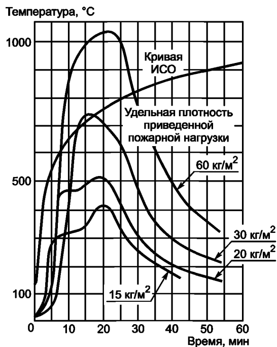
Рисунок 8 — Стандартная температурно-временная кривая пожара по соотношению (2) (кривая ИСО) и ее сравнение с зависимостями среднеобъемной температуры газа от времени, полученными при четырех полномасштабных экспериментальных испытаниях, характеризующимися одинаковым коэффициентом проемности по соотношению (3) и различной удельной плотностью пожарной нагрузки [8]
