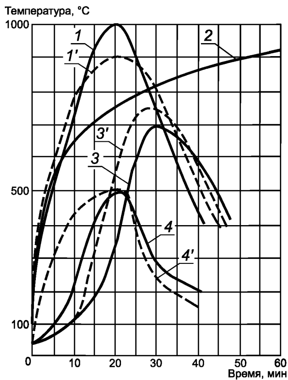
Рисунок 8а — Изменение среднеобъемной температуры при пожаре в помещениях 6 \times 6 \times 6 и 6 \times 6 \times 3 м 3 , \Pi = 25\% (см. [30])
