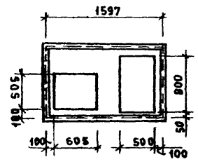
ОТВ. ДЛЯ УТЕПЛЕННОГО ЛЮКА 605 x 505 (h) ПО СЕРИИ 4.904-62
