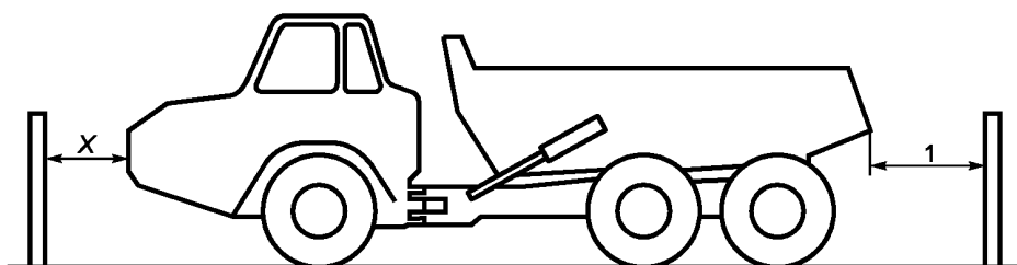
Рисунок А.5 — Землевоз с шарнирно-сочлененной рамой
