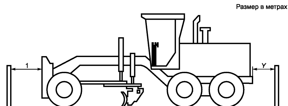
Рисунок А.6 — Грейдер
