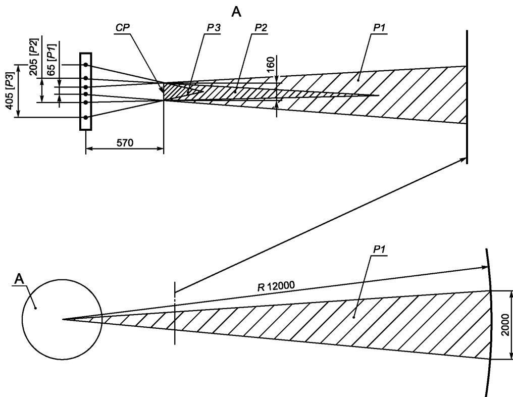
Рисунок 6 — Пример зависимости ширины непросматриваемой зоны от расстояния между лампами освещения
