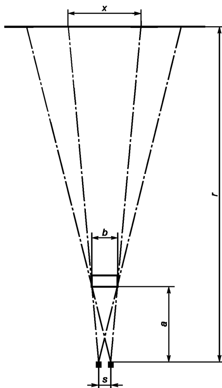
Рисунок 5 — Метод расчета для определения непросматриваемых зон
