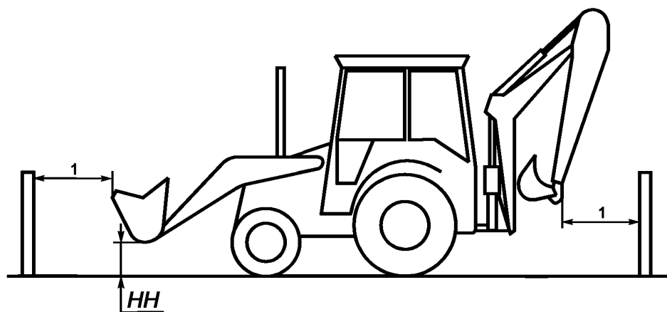
Рисунок А.2 — Экскаватор-погрузчик
