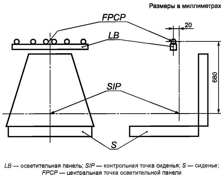
Рисунок 1 — Расположение источников освещения
