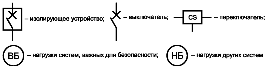
Рисунок 4 — Одна из резервированных частей системы питания СКУ
