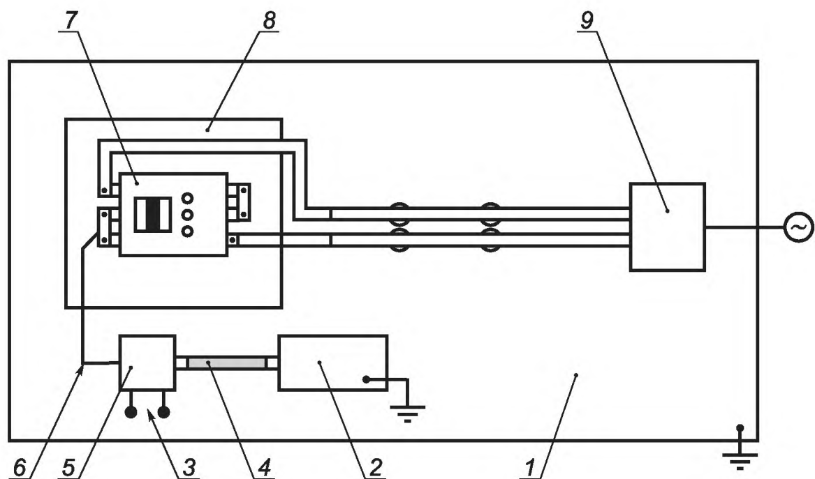
1 — заземляющая опора; 2 — высокочастотный генератор; 3 — сетевые выводы оставляют разомкнутыми; 4 — высокочастотное соединение; 5 — согласующее устройство М2; 6 — длина кабеля от 0,1 до 0,3 м; 7 — автоматический выключатель; 8 — изолирующая опора; 9 — трансформатор
