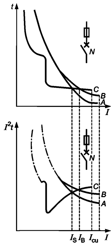
Рисунок А.1 — Рабочие характеристики координации по сверхтокам между автоматическим выключателем и предохранителем или резервной защитой, осуществляемой предохранителем
