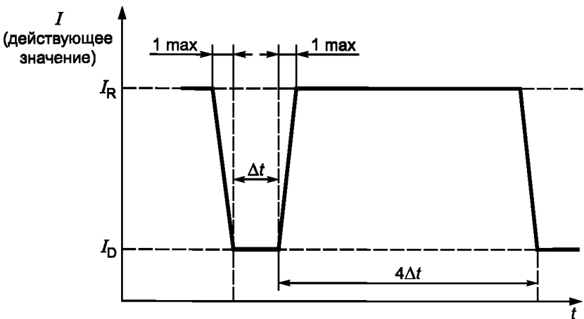
I_R — уставка тока; I_D — испытательный ток провала; \Delta t — время провала; 4\Delta t — время задержки
