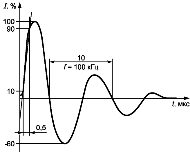
Рисунок В.4 — Волна тока 0,5 мкс/100 кГц
