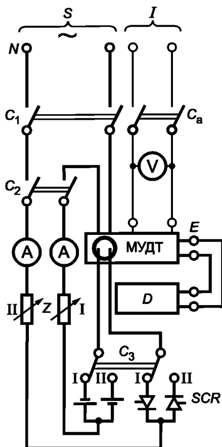
МУДТ со встроенным датчиком
