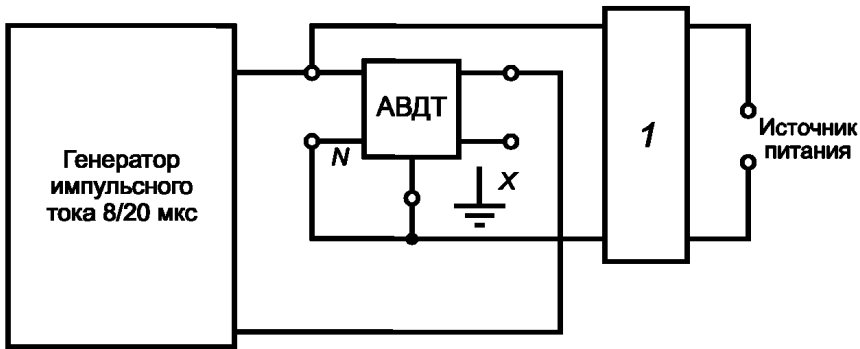
1 — фильтр; X — зажим заземления, если имеется, подсоединяемый к нейтральному зажиму, если он маркирован, или в отсутствие такой маркировки к любому фазовому зажиму; N — нейтраль
