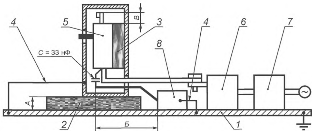
Размер A — (0,1—0,11) м; размер B — (0,9—1,0) м (полная длина кабеля); размер B — минимально возможный.
