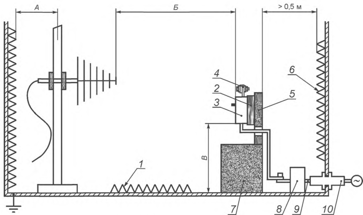
Размеры A , B и B — см. ГОСТ Р 51317.4.3.
