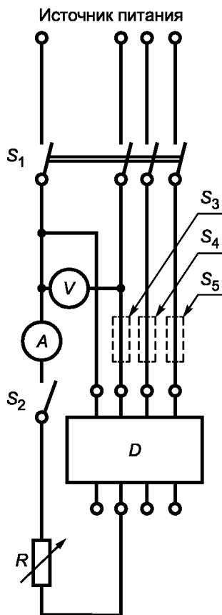
S_1 — многополюсный выключатель; S_2 — однополюсный выключатель; S_3, S_4, S_5 — однополюсные выключатели, отключающие фазы по очереди; D — испытуемый АВДТ; V — вольтметр; A — амперметр; R — регулируемый резистор
