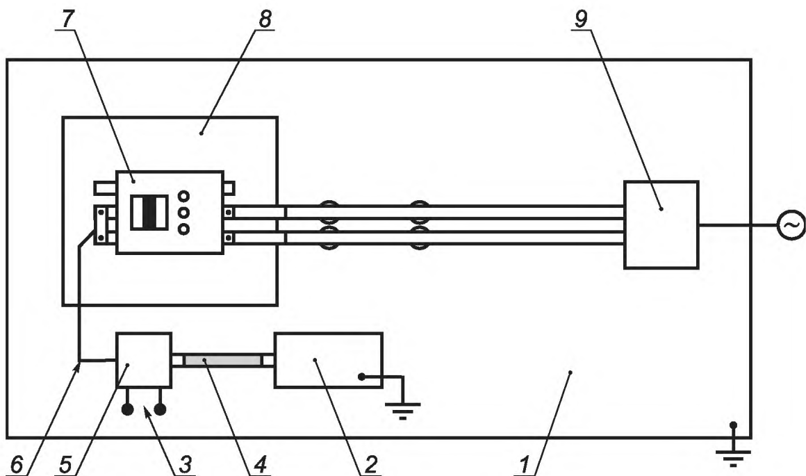
1 — заземляющая опора; 2 — высокочастотный генератор; 3 — сетевые выводы оставляют разомкнутыми; 4 — высокочастотное соединение; 5 — согласующее устройство M1 (M2 для рисунка F.22); 6 — длина кабеля от 0,1 до 0,3 м; 7 — автоматический выключатель (ОПИ); 8 — изолирующая опора; 9 — трансформатор
