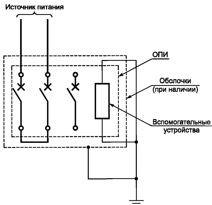
Рисунок Ф.2 — Испытательная цепь для проверки устойчивости к низкочастотным электромагнитным помехам и испытаний на помехоэмиссию по Ф.4.1.3, Ф.4.2, Ф.4.3, Ф.4.6, Ф.4.7.1, Ф.5.4 и Ф.6.2 для двух фазных полюсов, соединенных последовательно
