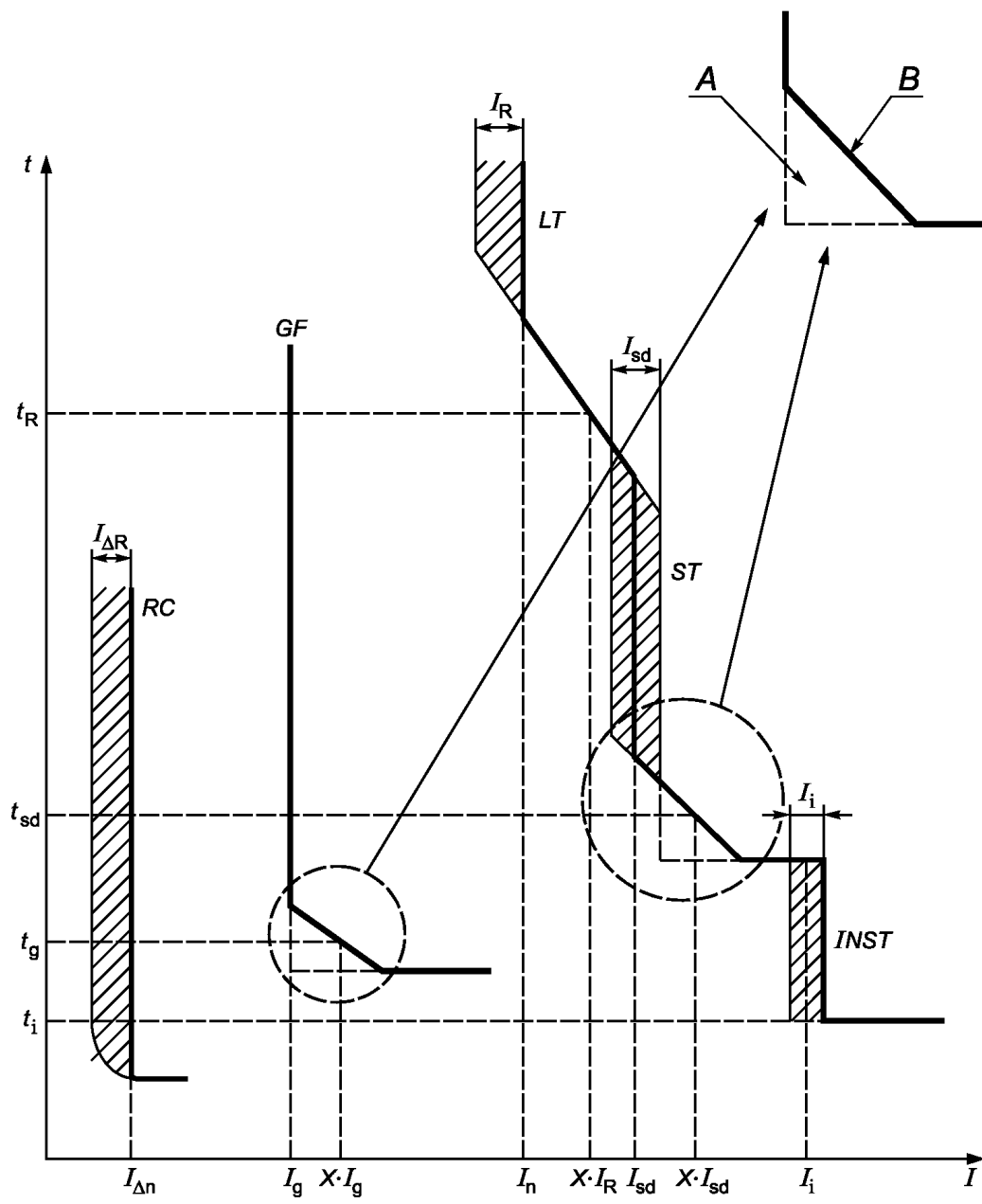
А — характеристика до I^2t ; В — характеристика I^2t ; RC — дифференциальный ток; GF — замыкание на землю; LT — длительное время; ST — коротковременно; INST — мгновенно
