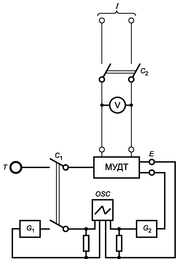
I — отдельный источник напряжения (при применении); V — вольтметр; C 1 — многополюсный выключатель; C а — вспомогательный выключатель; T — датчик; E — выходная цепь; G 1 , G 2 — генераторы; OSC — осциллограф
