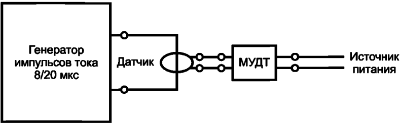
а) МУДТ с отдельным датчиком
