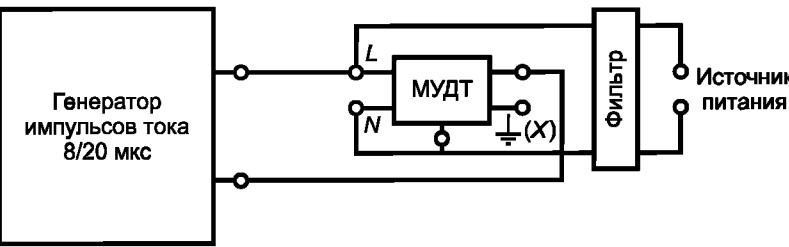
с) МУДТ выводного типа
