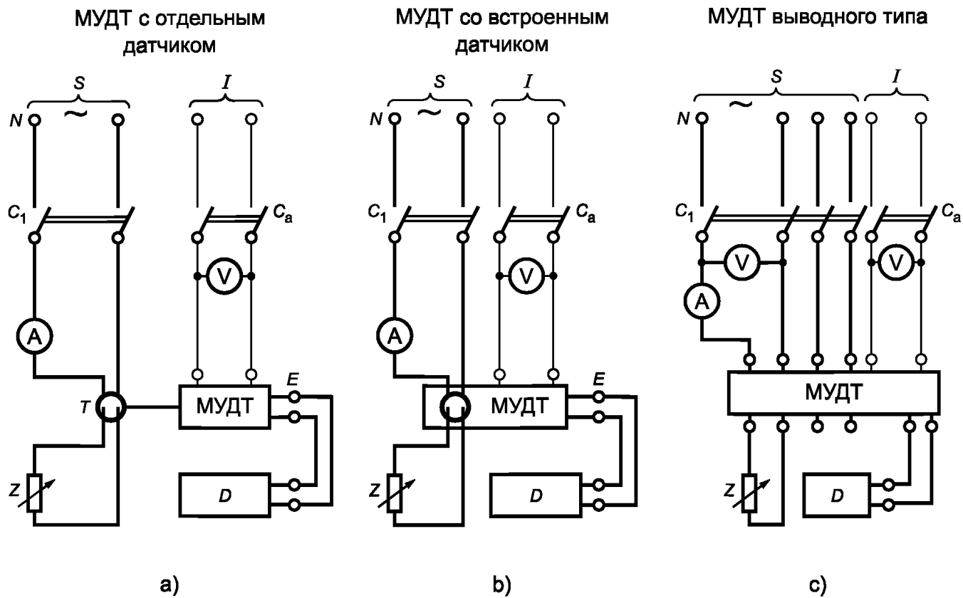
S — источник питания; I — отдельный источник напряжения (при применении); V — вольтметр; A — амперметр; C 1 — многополюсный выключатель; C a — вспомогательный выключатель; Z — регулируемое полное сопротивление; T — датчик; E — выходная цепь; D — прибор, регистрирующий изменение состояния; N — нейтраль
