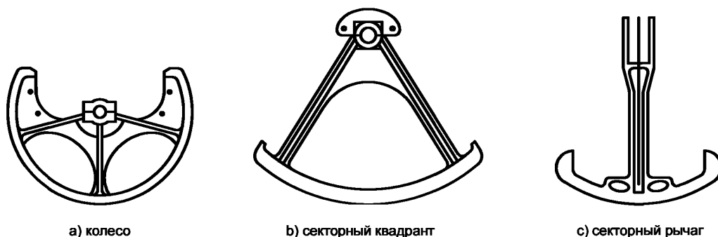
Рисунок 1 — Виды румпеля
