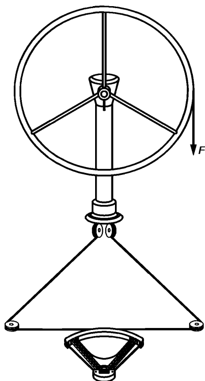
Рисунок 6 — Приложение касательной нагрузки
