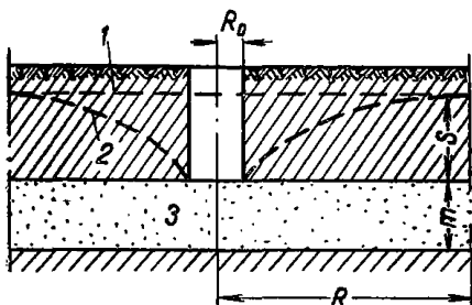
Рис. 2. Схема притока воды к широкому, не вытянутому в длину, котловану, вскрытому своим дном напорный водоносный пласт:
