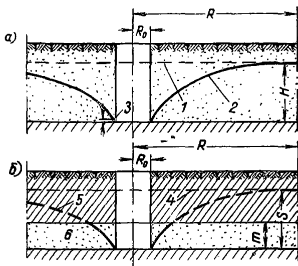
Рис. 1. Схема притока воды к широкому, не вытянутому в длину, котловану совершенного типа: а) в безнапорных водах; б) в смешанных условиях
