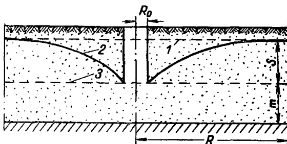
Рис. 3. Схема притока воды к широкому, не вытянутому в длину, котловану несовершенного типа при работе его в безнапорных водах:
