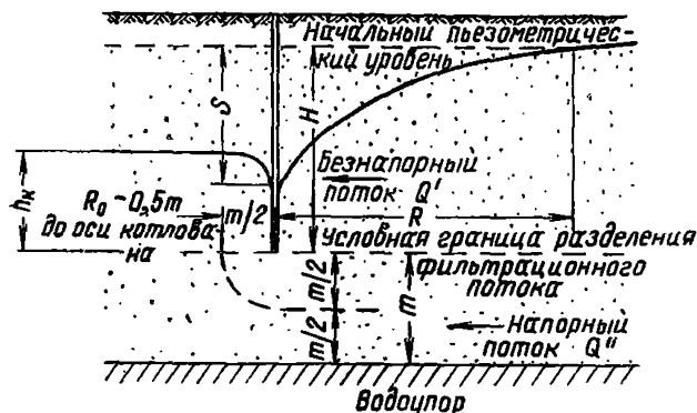
Рис. 3. Расчетная схема водопонижительной установки несовершенного типа
