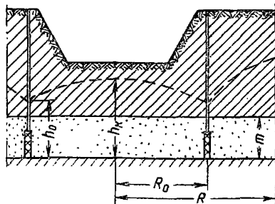
Рис. 2. Схема водоопонижения при разработке котлована в условиях напорного водоносного горизонта
