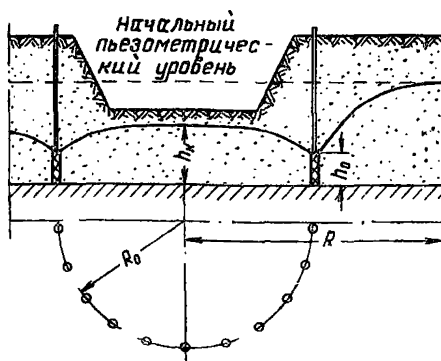
Рис. 1. Схема водоопонижения при разработке котлована в безнапорных водах
