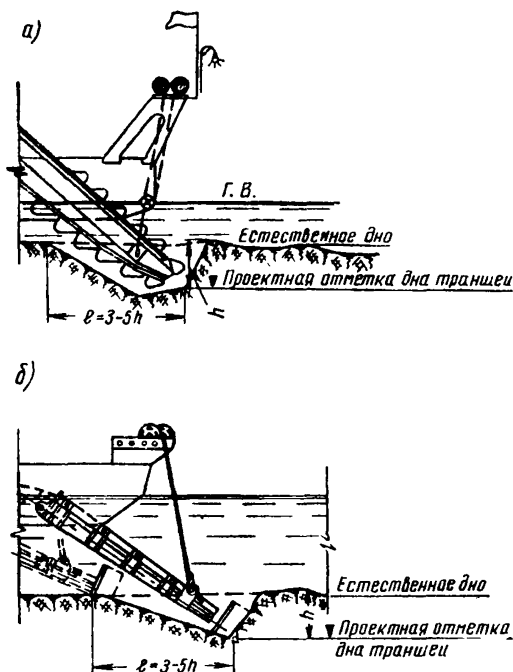
Рис. 2. Схема врезки в траншею земснаряда:
