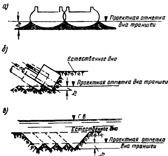
Рис. 1. Схемы разработки траншей земснарядами:
