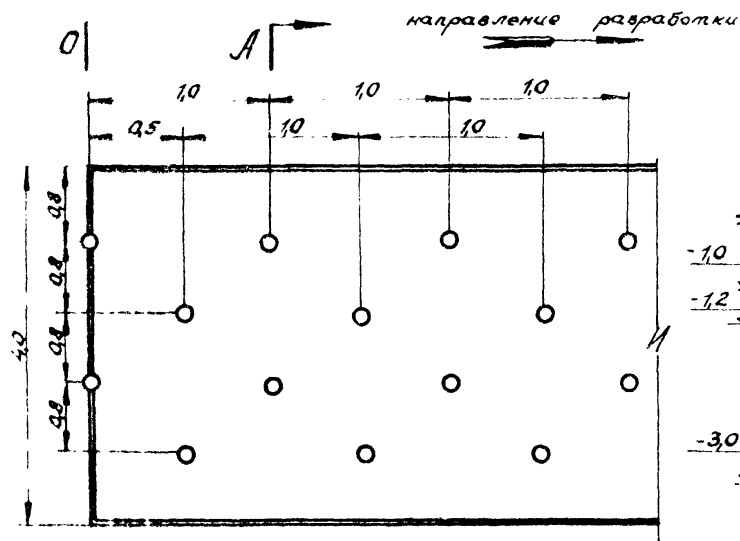
рис. 4 Схема расположения шпуров при проходке траншеи
