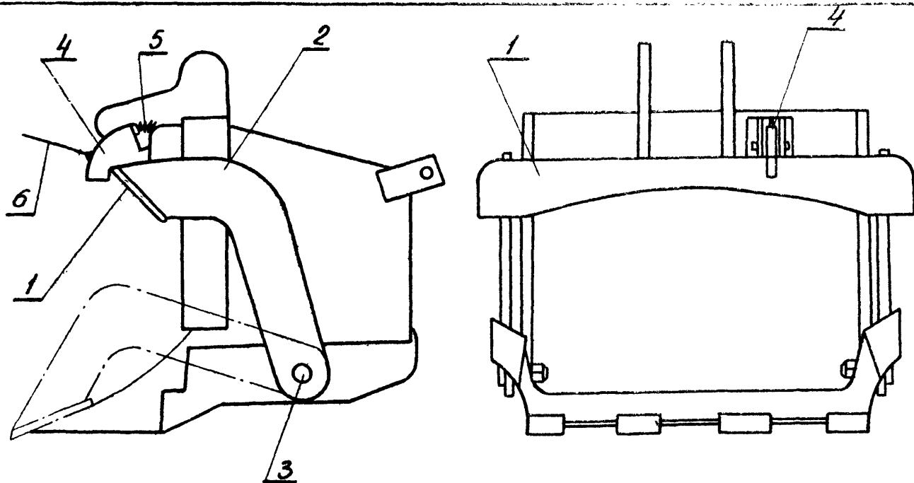
Рис.2 Струг для зачистки дна траншеи экскаватором.
