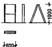
38 Мольберт низ- кий складной
