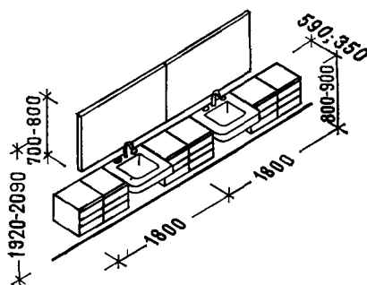
6 Туалет парикмахерский с умывальником
