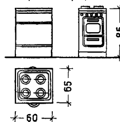
19 Плита бытовая электрическая четырёхконфорочная
