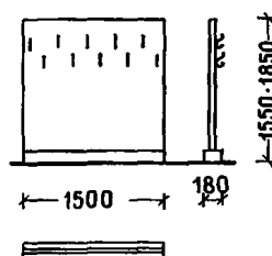
13 Вешалка для верхней одежды
