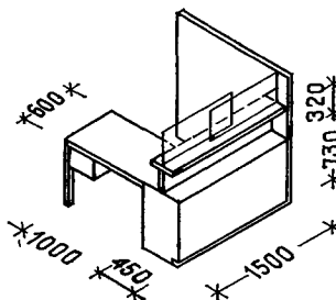
1,2 Барьер почты со столом-приставкой
