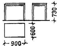
4 Стол письменный двухтумбовый
