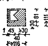
Шкаф медицинский двухстворчатый
