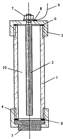
Рисунок 1 — Принципиальная схема конструкции переносного медно-сульфатного электрода сравнения
