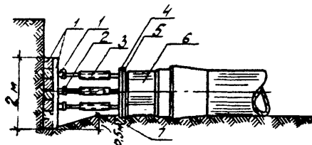
Рис.2 Упор в ненарушенный грунт.
