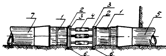
Рис.3. Упор в уложенный трубопровод
