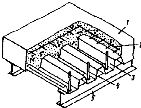
Рис. 5.3 Конструкция СБП
