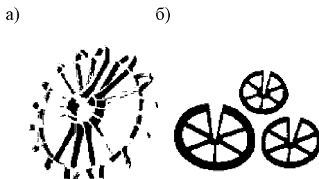
Рис. 5.6 Фиксаторы арматуры
