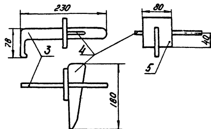
Крюк с клиновым запором
