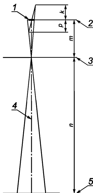
1 — ЭФФЕКТИВНОЕ ФОКУСНОЕ ПЯТНО; 2 — ОПОРНАЯ ПЛОСКОСТЬ; 3 — входная плоскость диафрагмы; 4 — ОПОРНАЯ ОСЬ; 5 — ПЛОСКОСТЬ ПРИЕМНИКА ИЗОБРАЖЕНИЯ
