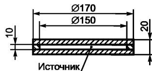
Рисунок 1 — Кювета
