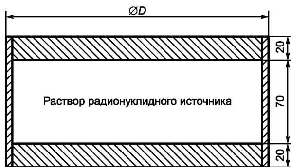
Рисунок 3 — Однородный источник
