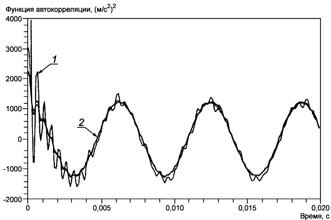
1 — СПУ: 0,01 g_n^2 / \text{Гц} ; 2 — СПУ: 0,005 g_n^2 / \text{Гц}
