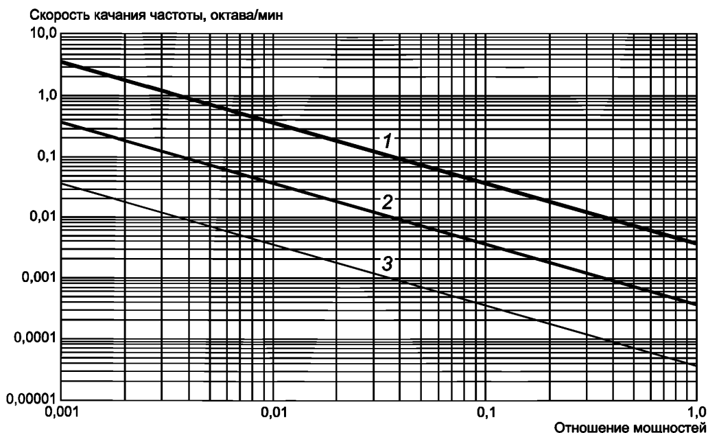
Рисунок 5 — Рекомендуемая скорость качания частоты в зависимости от отношения мощностей для разных значений E_{sor}
