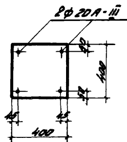
БЕТОН М7-300
