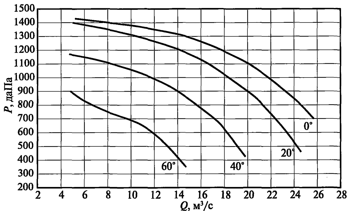
Рис. 2. Аэродинамическая характеристика вентилятора УВЦГ-9
