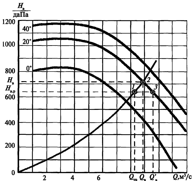
Рис. 1. Определение допустимой величины подсвеживания отсасываемой метановоздушной смеси
