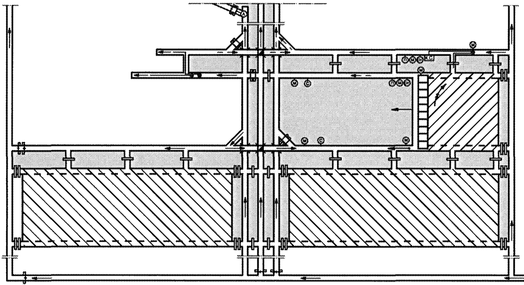
Рис. 5. Схема проветривания выемочного столба с отводом метановоздушной смеси по выработанному пространству подземной ГОУ с ее поэтапным перемонтажом вслед за продвижением очистного забоя
