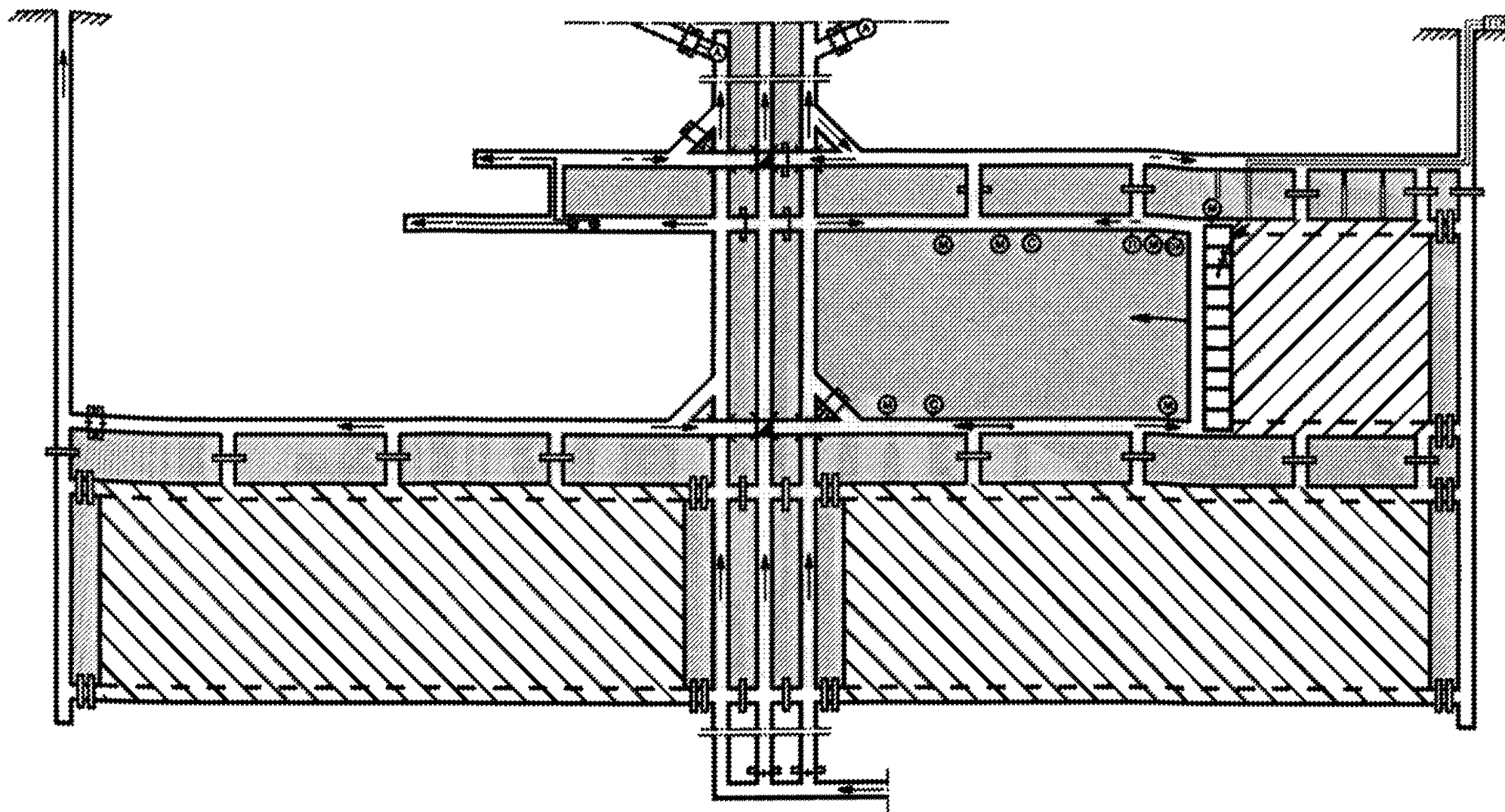
Рис. 4. Схема проветривания выемочного столба с отводом метановоздушной смеси по выработанному пространству и скважине (сбойке) в межлавном целике в газоотсасывающий (дегазационный) трубопровод и на поверхность ГОУ
