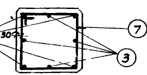
Сечение II-II
