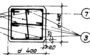
Сечение II-II
