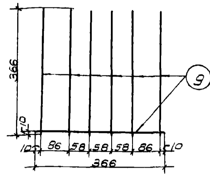
Гребенка
