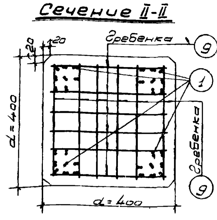
Гребенка
