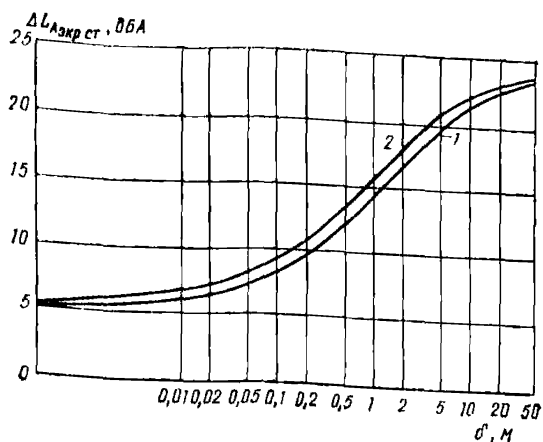
Рис. 6. Графики для определения снижения уровня звука экраном-стенкой
