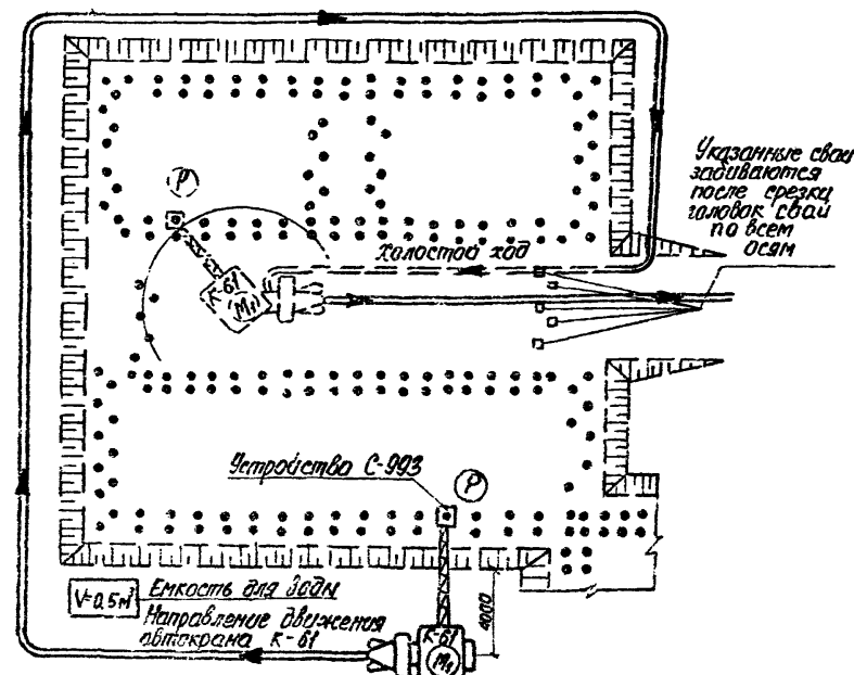
Рис.13. СХЕМА ОРГАНИЗАЦИИ РАБОЧЕГО МЕСТА ПРИ СРЕЗКЕ ГОЛОВКИ СВАЙ
