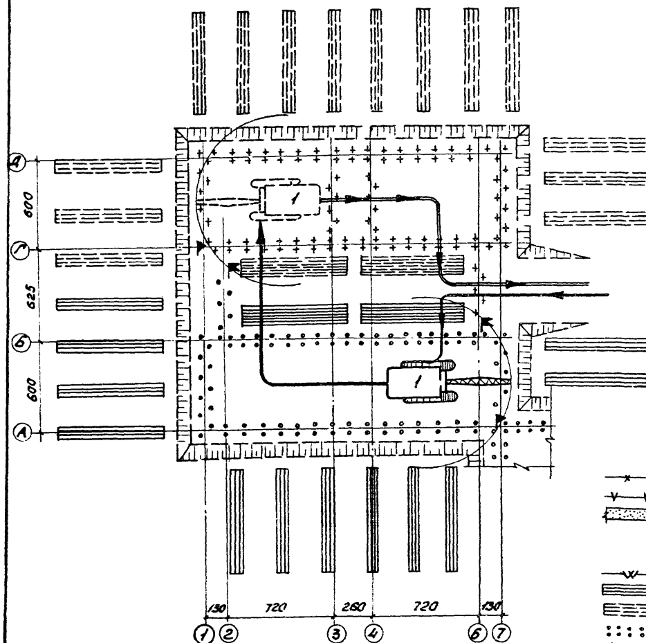
Рис.2. СХЕМА ПРОИЗВОДСТВА РАБОТ ПО ЗАБИВКЕ СВАЙ НА ЗАХВАТКЕ-СЕКЦИИ ЖИЛОГО ДОМА СЕРИИ Ir-447C-26/65 КОПРМ НА БАЗЕ ЭКСКАВАТОРА
