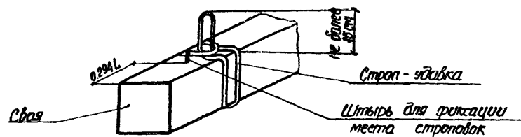
Рис.7. СТРОПОВКА СВАЙ
