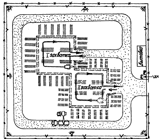
Рис.3. СХЕМА ПРОИЗВОДСТВА РАБОТ НА ОБЪЕКТЕ
