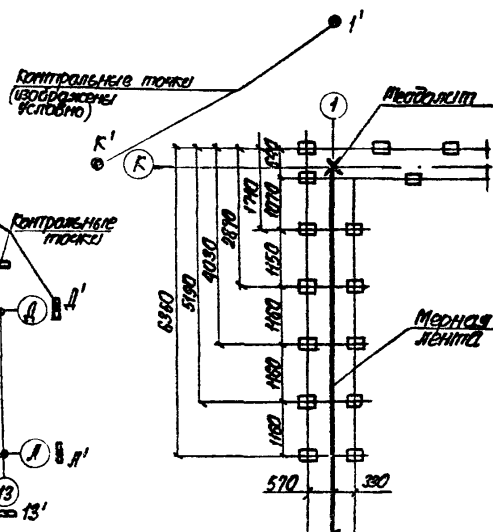
Рис.5. РАЗБИВКА СВАЙНОГО РЯДА
