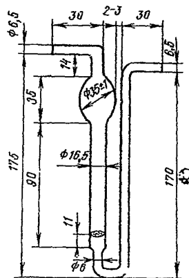
Рис. 3. Поглощающий прибор с пористой пластинкой
