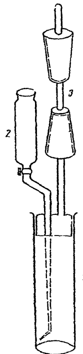
Рис. 4. Прибор для получения мышьяковистого водорода: 1 — пробирка с прилифированной пробкой; 2 — делительная воронка; 3 — индикаторная трубка Бальской
