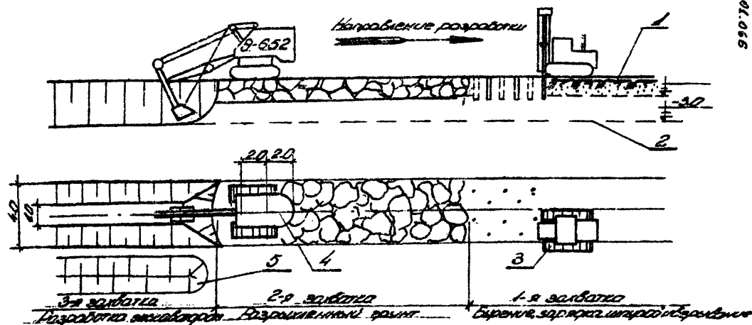
рис. 3 Схема разработки траншеи при рыхлении мерзлого грунта взрывчатым способом
