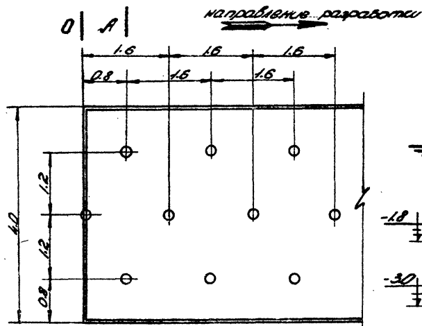
0 | А | рис. 5 Система расположения шпуров при проходке траншеи
