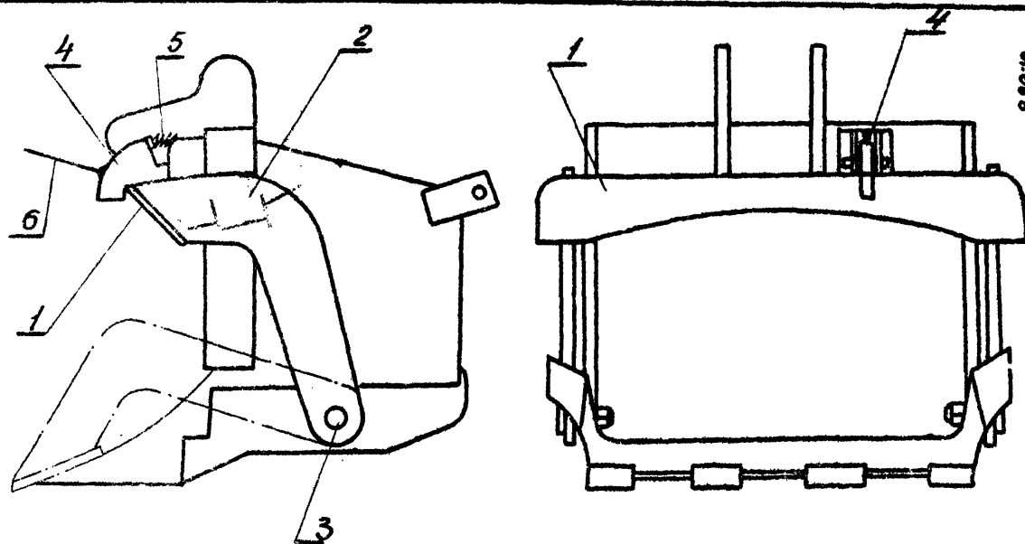
Рис.2 Струа для зачистки дно траншей экскаватором. 1-Нож струа; 2-упорные штанги; 3-цапга; 4-заток-защелка; 5-пружина; 6-тросик
