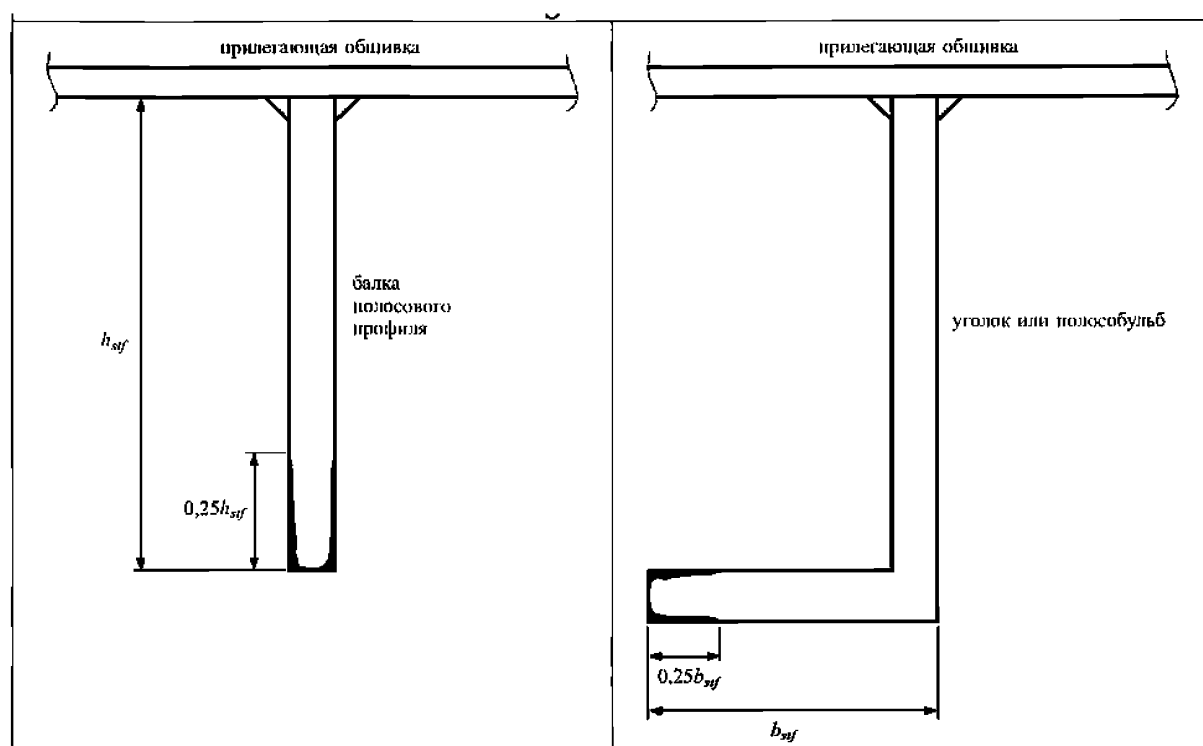
Рис. 1.2.1-5 Коррозия кромок
