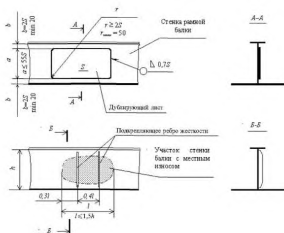
Рис. 5.2.4.2 Подкрепление участка балки набора
