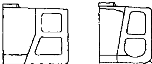
Рис. 2.2.6 Типовые сечения мидель-шпангоута рудовоза
