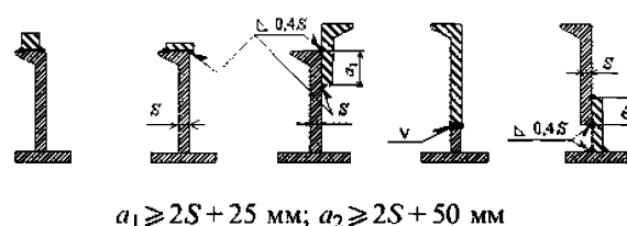
Рис. 5.2.4.1-1 Подкрепления балок набора:
