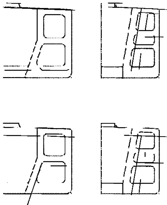
Рис. 2.2.7.2 Типовые сечения мидель-шпангоута нефтерудовоза
