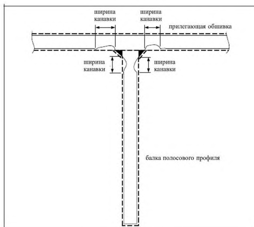
Рис. 1.2.1-4 Канавочный износ
