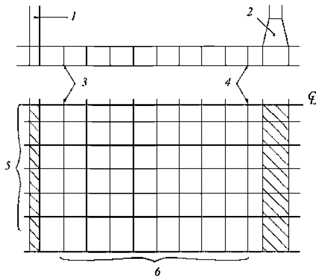
Рис. 5.10.3 Донные конструкции грузового трюма
