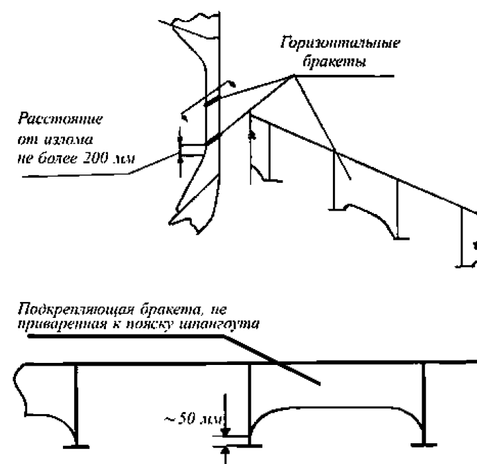
Рис. 5.12.3.3.1 Подкрепляющие brackets
