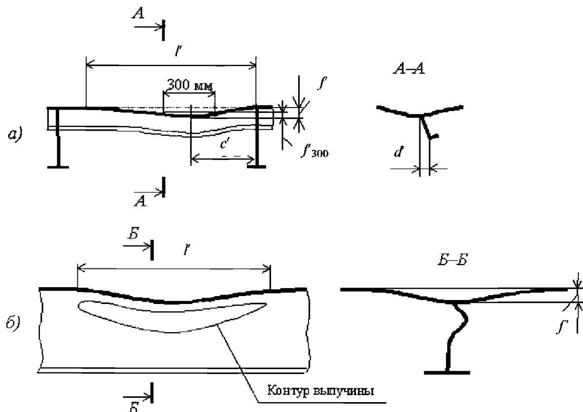
Рис 3.3.4.2 Измерение параметров вмятин:
