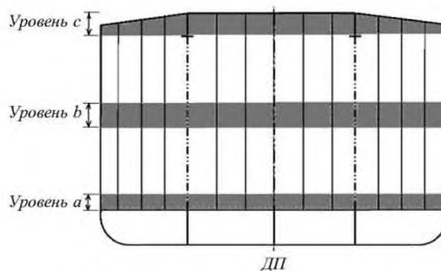
Рис. 7.2.3.2-4 Уровни a, b и c детального освидетельствования поперечной переборки грузового трюма, не имеющего твиндека, на судах, предназначенных для перевозки сухих генеральных грузов
