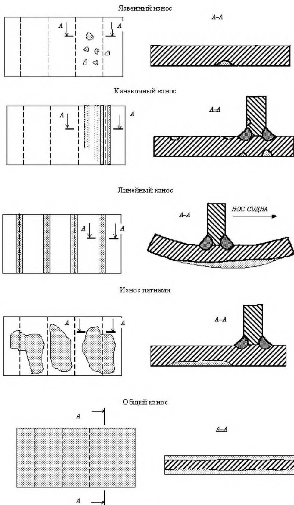
Рис. 1.2.1-2 Виды износов
