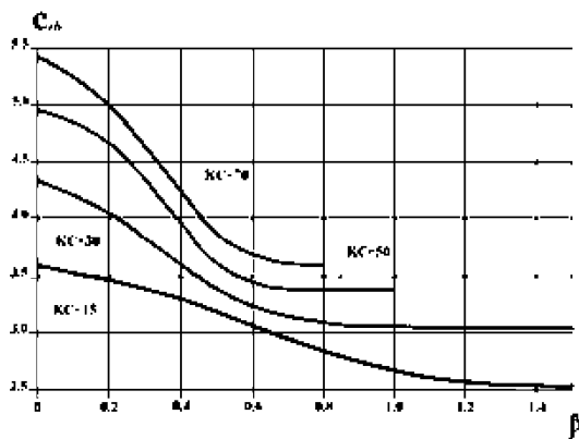
Рис. 9-2 Коэффициент c_{ib} в зависимости от коэффициента \beta
