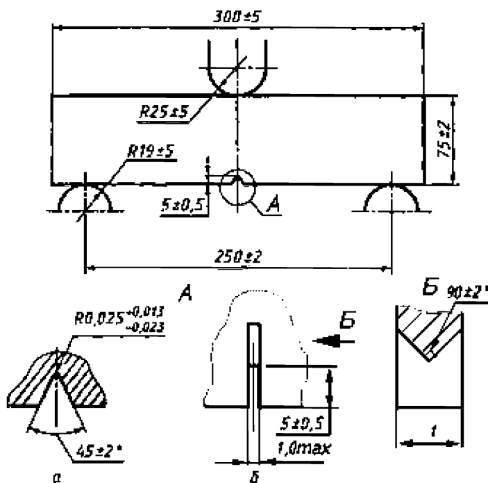
Рис. 1.2 Образец и оснастка для испытаний ( t – толщина)
