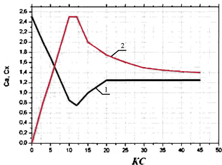
Рис. 2.5 Зависимости коэффициентов скоростного c_x (1) и инерционного c_a (2) сопротивления от числа Кюлегана-Карпентера KC
