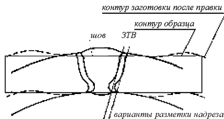
Рис. 5.4.4.3 Разметка образцов из трубы
