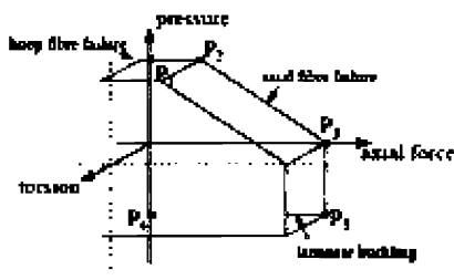
Рис. 4 Общая поверхность разрушения трубы райзера из ПКМ, нагруженной внешним давлением, осевой силой и крутящим моментом.
