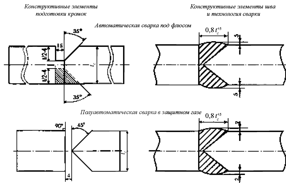
Рис. 5.2.4.2 Сварные соединения для испытаний на свариваемость
