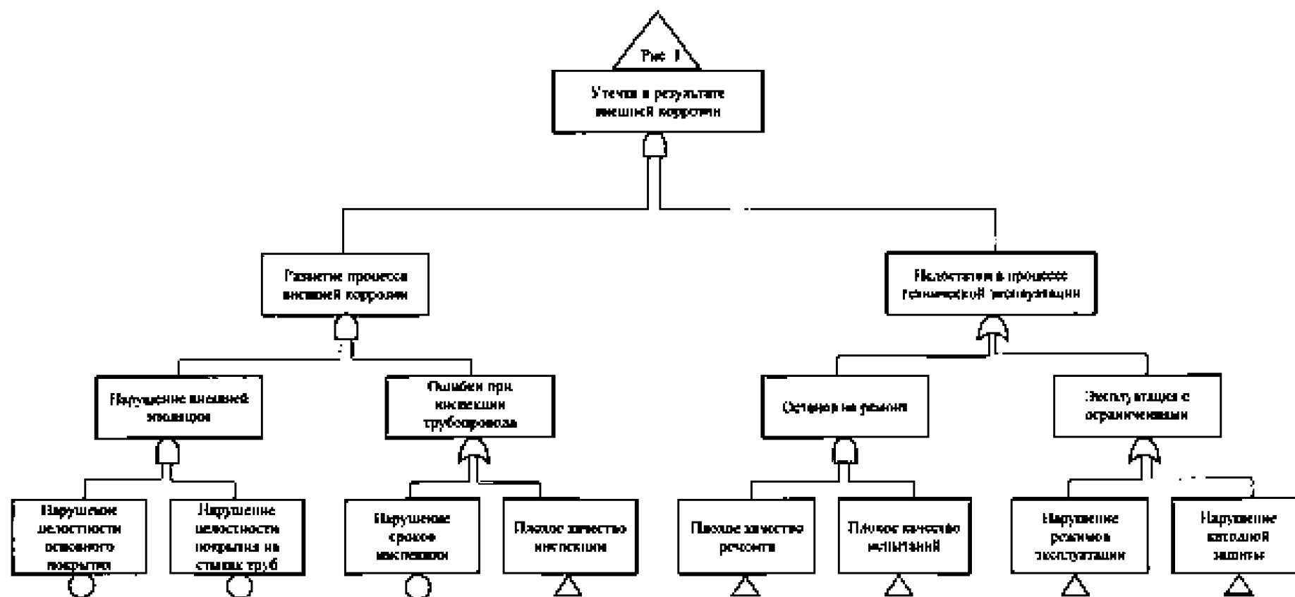
Рис. 2 Дерево отказов для аварии, связанной с внешней коррозией подводного трубопровода
