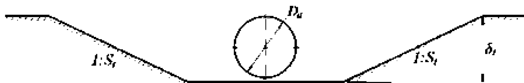
Рис. 4 Схема трубопровода, расположенного в открытой траншее
