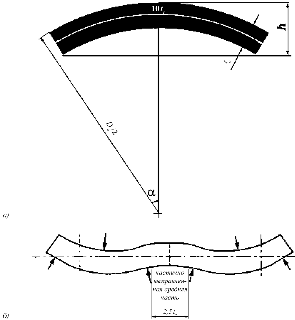
Рис. 2.1 Правка поперечных заготовок из трубы
