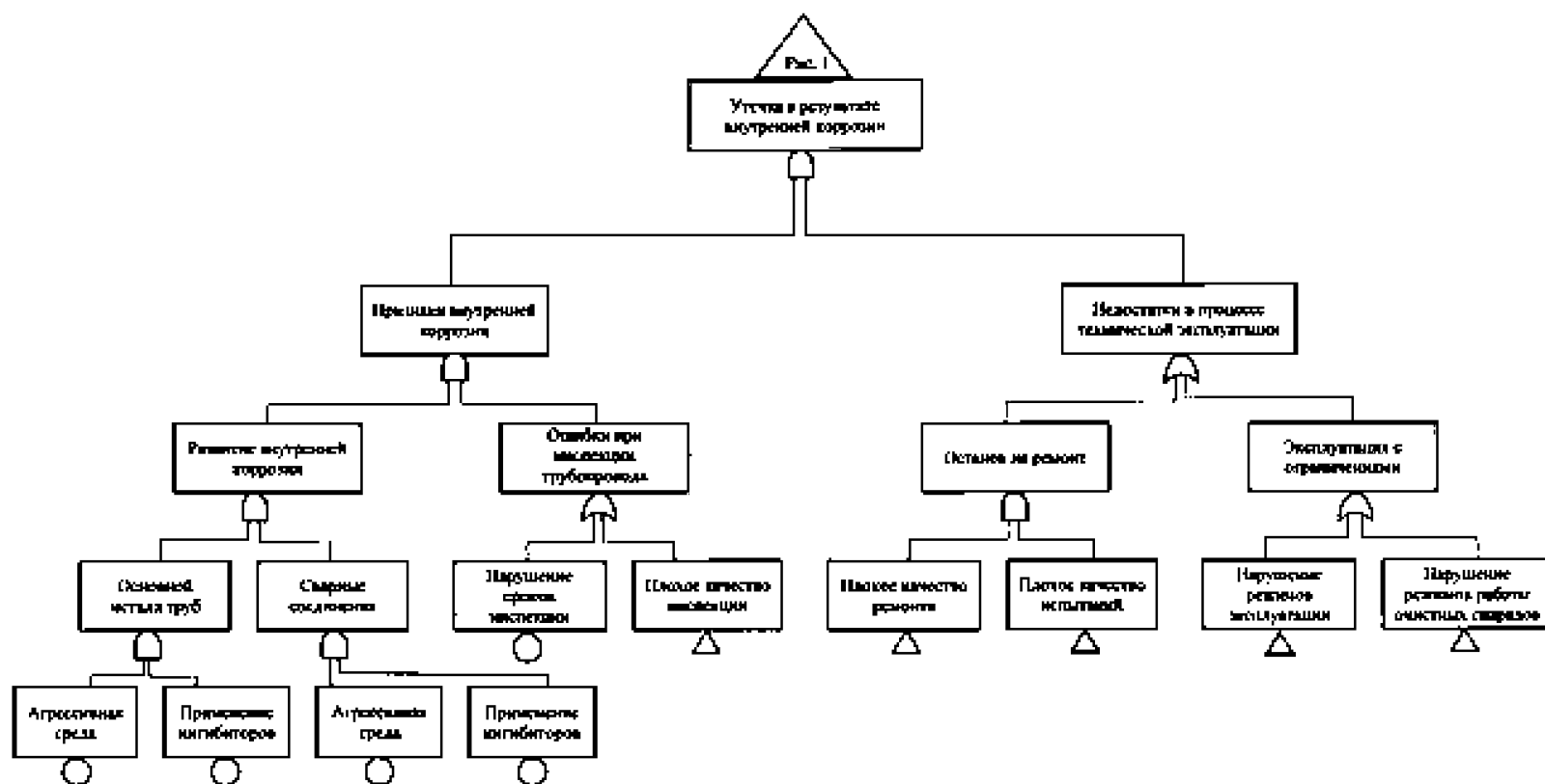
Рис. 3 Дерево отказов для аварии, связанной с внутренней коррозией подводного трубопровода
