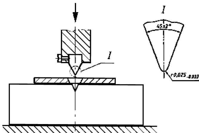
Рис. 1.3 Схема приспособления для прессования надрезов
