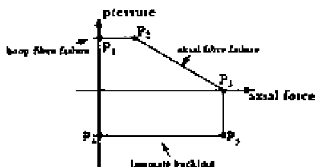
Рис. 3 Поверхность разрушения трубы райзера из ПКМ, нагруженной внутренним давлением и осевой силой.
