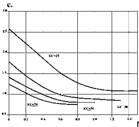
Рис. 9-3 Коэффициент c_v в зависимости от коэффициента \beta
