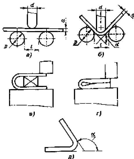
Рис. 3.1 Схема испытаний на изгиб
