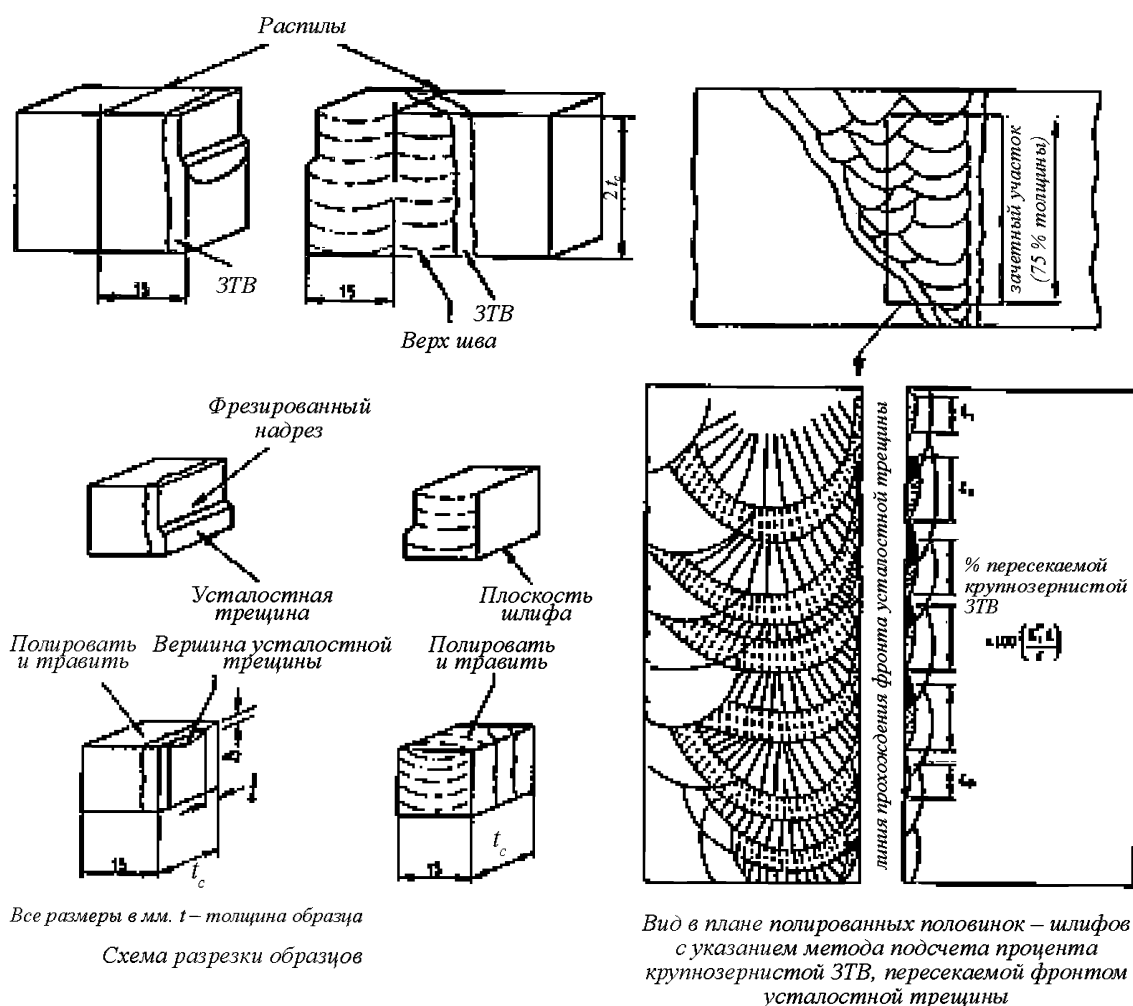
Рис. 5.4.4.8 Порядок металлогрифического исследования после испытания
