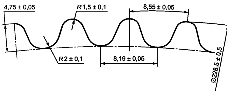
Рисунок 1 — Профиль гофрирующих дисков и основные размеры (мм)
