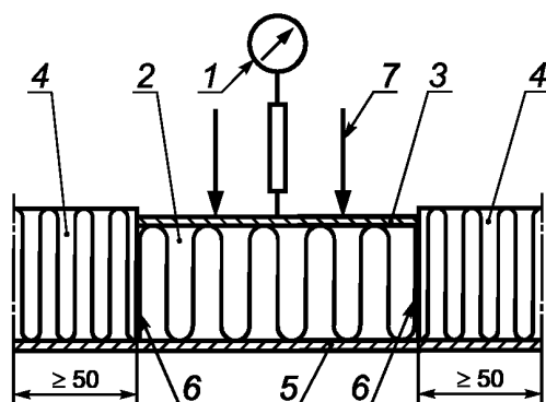
1 — средство измерений деформации образца; 2 — образец; 3 — опорная пластина для груза; 4 — боковая изоляция; 5 — нагреваемая пластина, термостатируемая с погрешностью до 0,5°C; 6 — зазор; 7 — испытательная нагрузка
