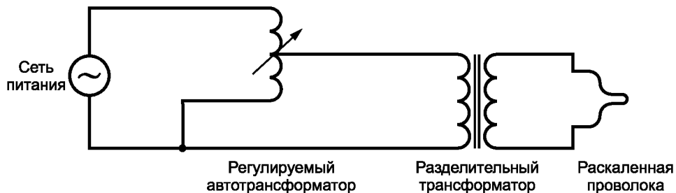
Рисунок 2 — Испытательная цепь
