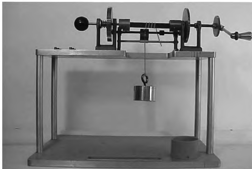
Рисунок 4 — Пример намоточного устройства
