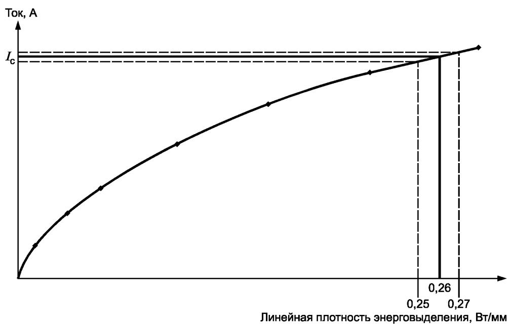
Рисунок А.2 — Калибровочная кривая
