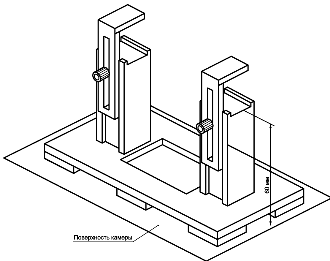
Рисунок 3 — Пример зажимного приспособления
