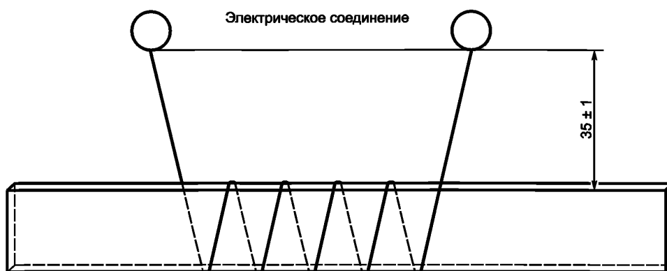
Рисунок 2 — Пример намотки проволоки на испытуемый образец
