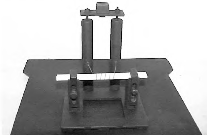
Рисунок 1 — Пример монтажа испытательного зажимного приспособления
