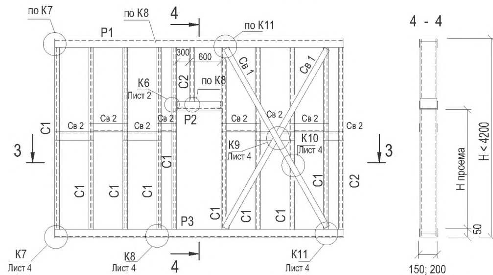
Фрагмент 1 каркаса с дверным проемом
