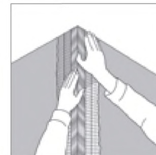
Рис. 20. Армирование углов
