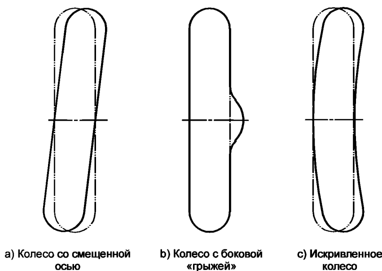
Рисунок 8 — Некоторые боковые отклонения колес
