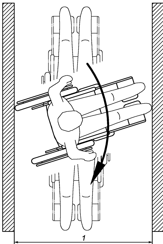
Рисунок 9 — Ширина вращения
