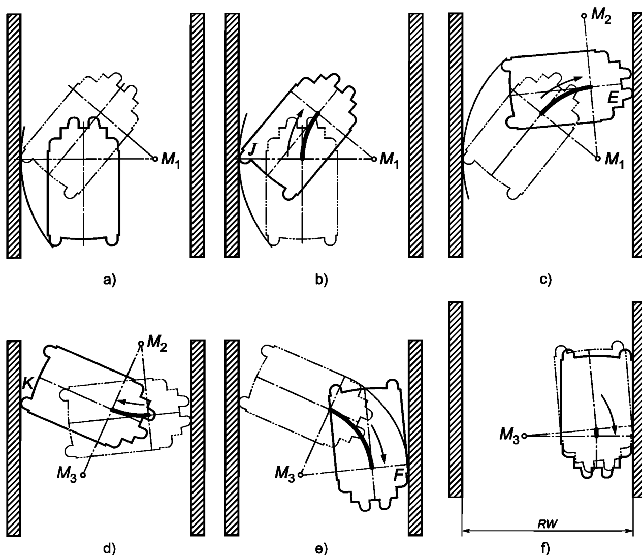
а) — ф) — последовательность маневров; F, E, J, K — точки, которые соприкасаются со стенами; M_1 - M_3 — центры трех маневров разворота; RW — ширина разворота
