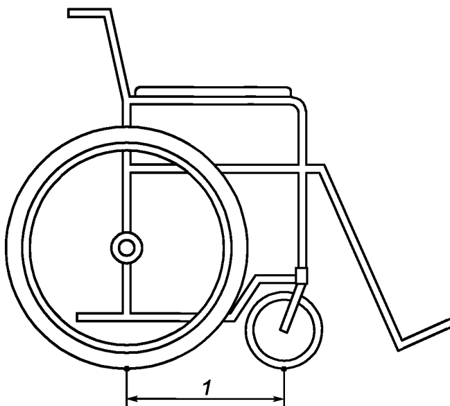
Рисунок 20 — Колесная база
