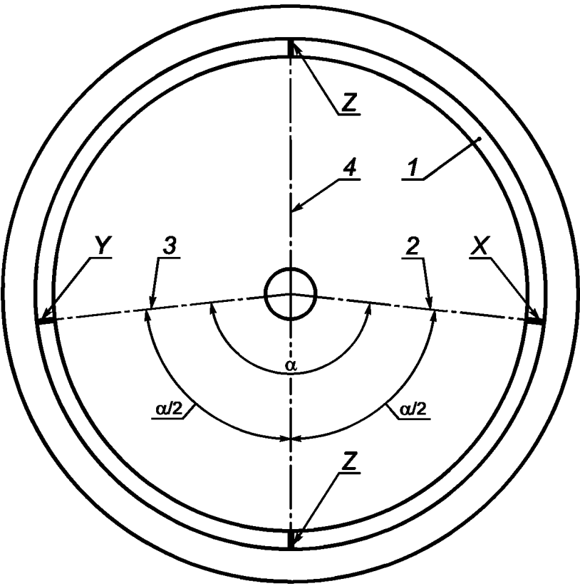
X — наиболее удаленная боковая точка обода; Y — наименее удаленная боковая точка обода; Z — нейтральное поперечное отклонение обода; 1 — лицевая сторона обода; 2 — радиус, проходящий через точку X; 3 — радиус, проходящий через точку Y; 4 — линия, делящая пополам угол между радиусами 2 и 3; α — угол между радиусами 2 и 3
