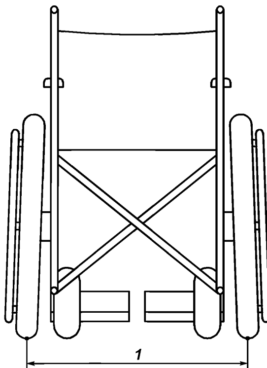
Рисунок 12 — Колея задних колес (пример)
