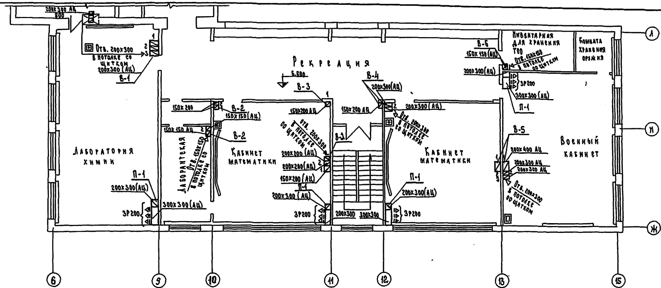
БЛОК „А“ 3 ий ЭТАЖ
