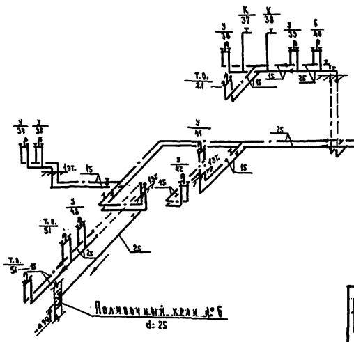
Схема водоснабжения корпусов "А" и "В"
