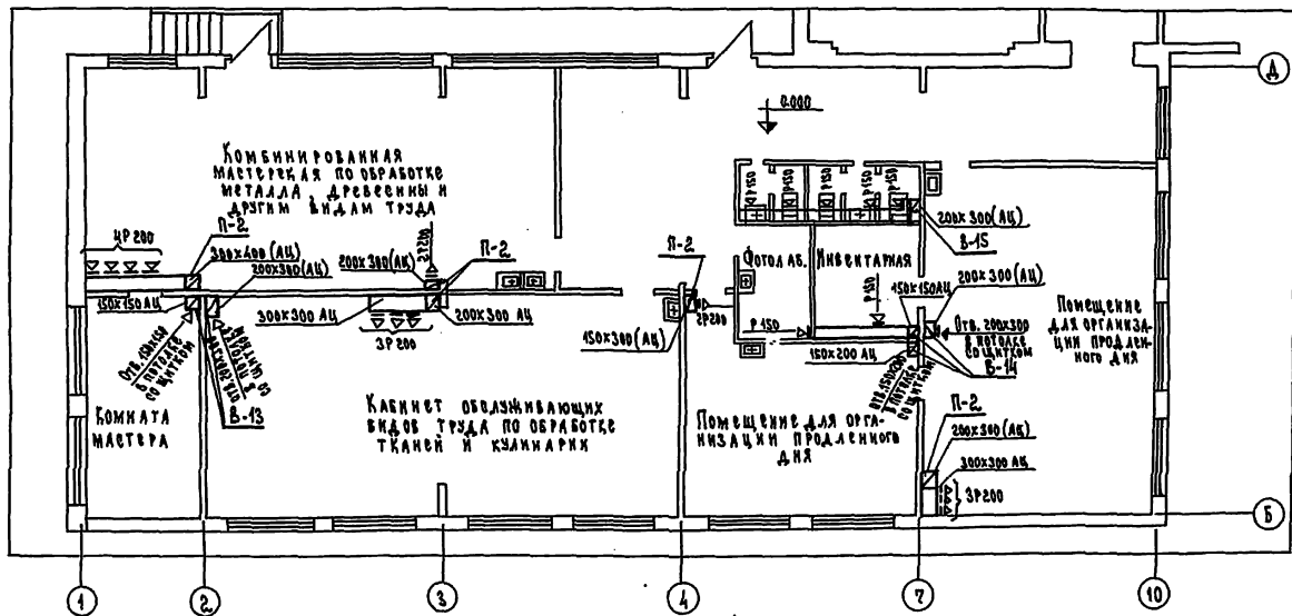
БЛОК „В“
