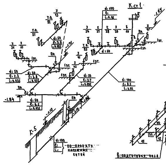
Схема канализации корпуса "В"
