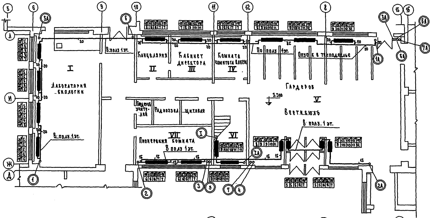
План 1 этажа
