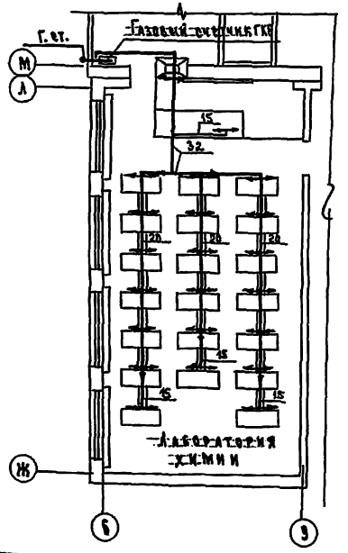
Выкопировка из плана 3 го этажа
