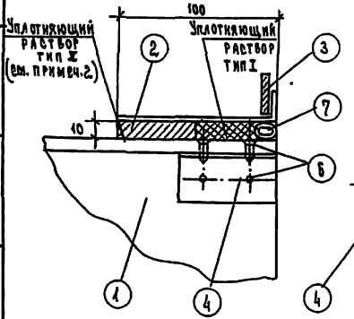
Узел I
