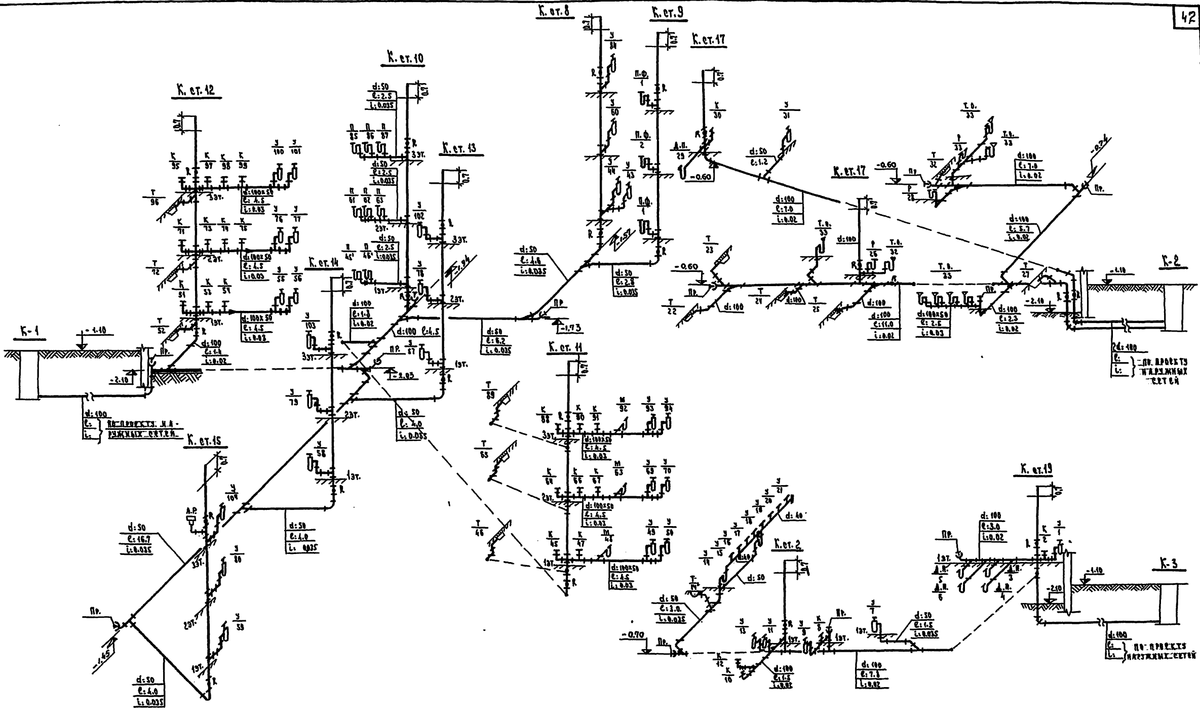
Схема канализации корпуса А.Б.
