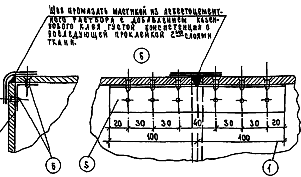
Узел II
