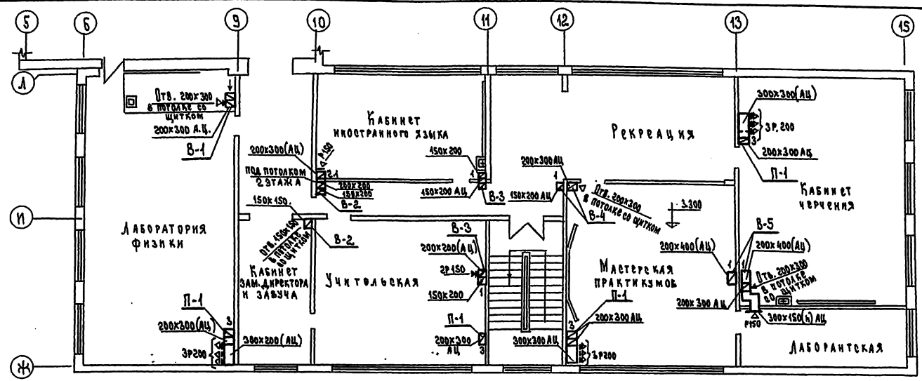
План 2 эт.
