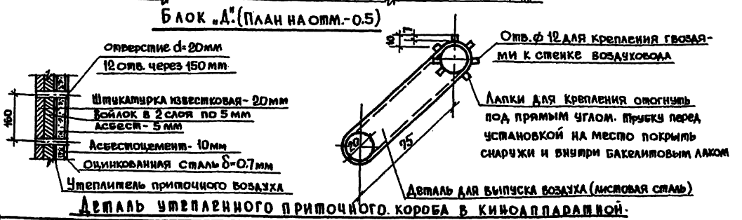
Вентиляция. Блоки "Г" и "А". Планы.
