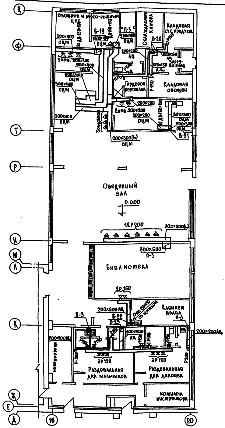
Блок "Г"
