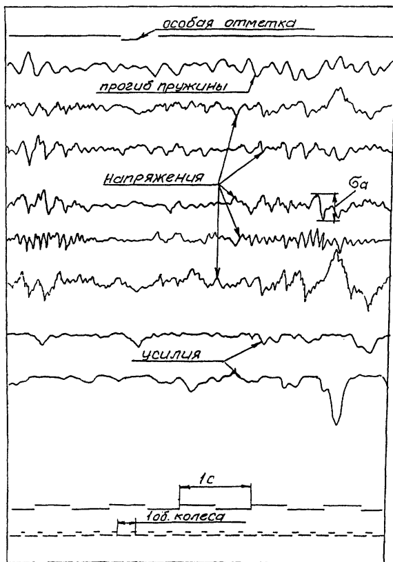
Рисунок 5 - Образец осциллограммы
