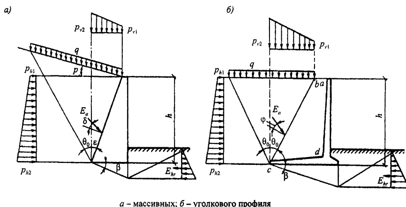
Рисунок 1 – Расчетные схемы подпорных стен
