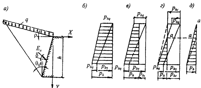
a – на стену; б – при отсутствии сцепления p_{hc} = 0 ; в – при p_{hc} < p_{hq} ; з – при p_{hc} \geq p_{hq} ; д – заменяющая (расчетная) эпюра
