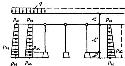
Рисунок 2 – Расчетная схема поперечной рамы подвала
