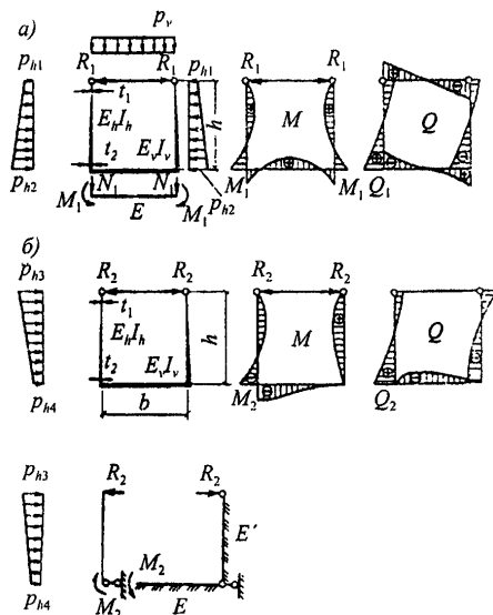
а – симметричное нагружение; б – одностороннее нагружение
