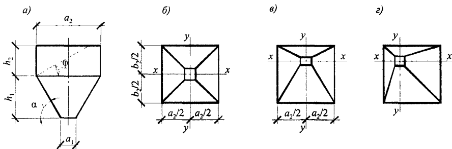
а – схема бункера; б – симметричный пирамидальный бункер; в – частично симметричный пирамидальный бункер; г – несимметричный пирамидальный бункер
