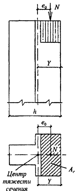
Рисунок 5 – Внецентренное сжатие
