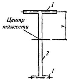
1 – простенок продольной стены; 2 – поперечная стена
