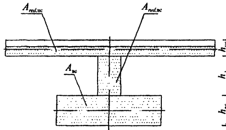
Рисунок 10 – Приведенное сечение рассчитываемого фрагмента стены
