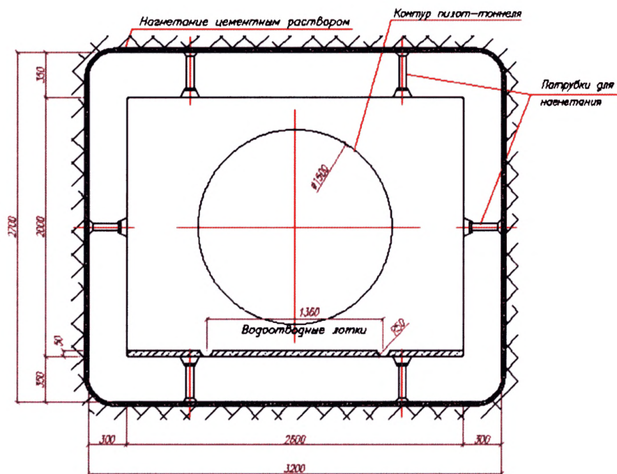
Рисунок 1 - Поперечное сечение цельносекционной обделки
