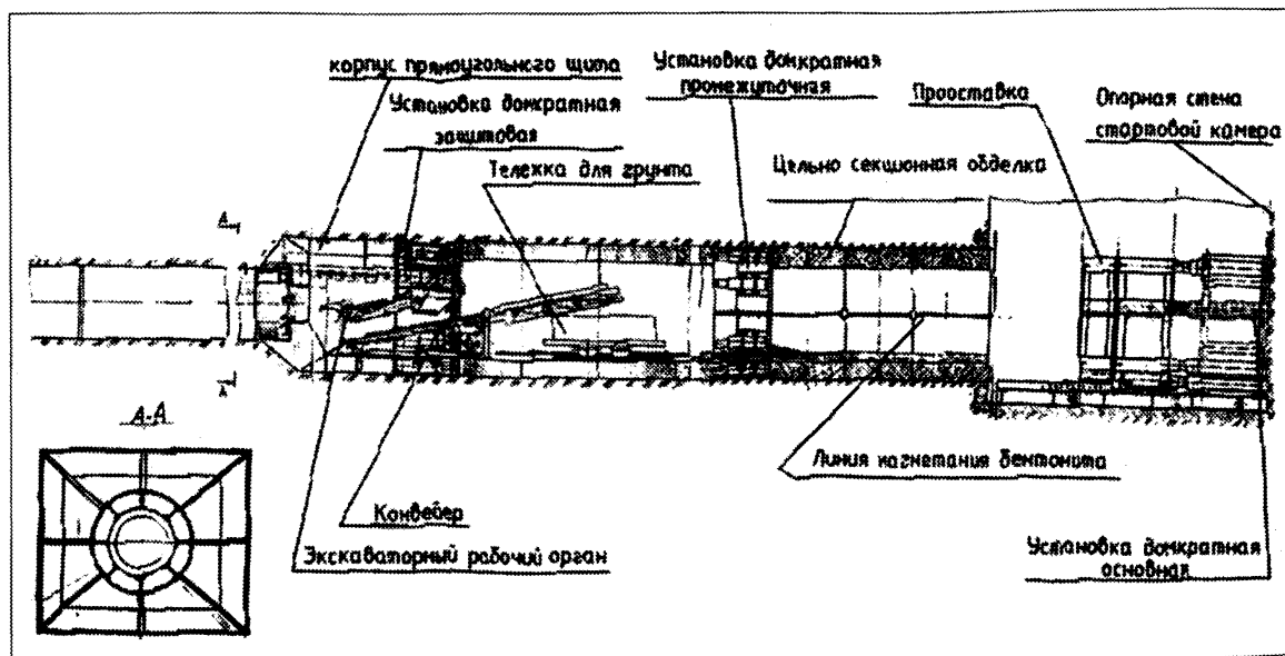
Рисунок 2 – Принципиальная конструкция прямоугольного тоннелепроходческого комплекса
