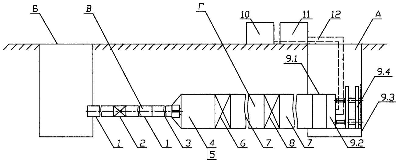
Рисунок 3 – Схематическая структура комплекса
