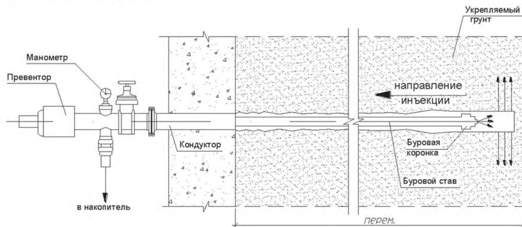
Рисунок В.2 – Оборудование скважин превенторным устройством и методы инъекции
