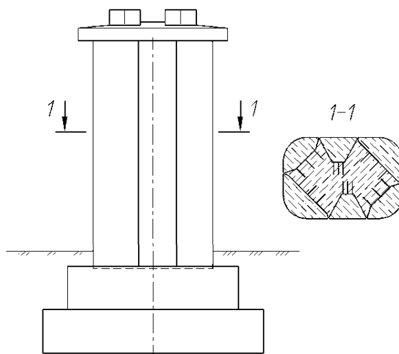
Рисунок 8.2 – Опоры с вертикальными железобетонными контурными блоками
