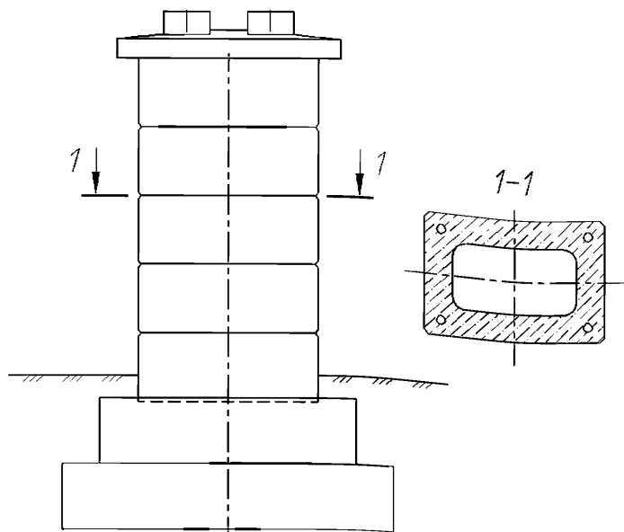
Рисунок 8.3 – Опоры с пустотелыми горизонтально располагаемыми блоками
