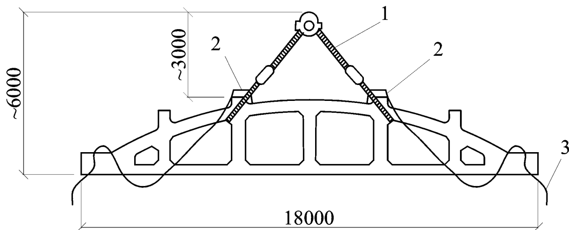
1 – строп; 2 – пружинный замок Пр8; 3 – канат для расстроповки
