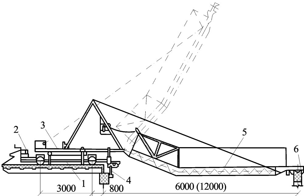
Рисунок 11 – Инвентарная распорка
