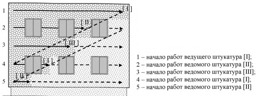
Рисунок 7 – Горизонтально-нисходящая схема устройства декоративно-защитного финишного слоя
