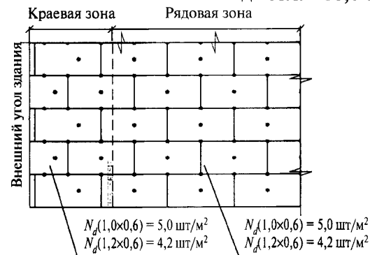
Рисунок 4 – Схемы установки тарельчатых дюбелей
