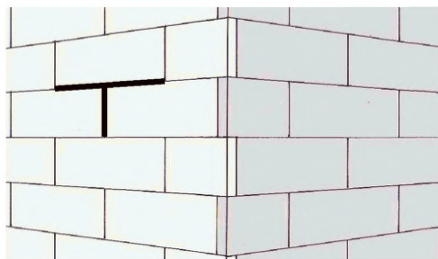
Рисунок 3 – Схема исполнения зубчатого зацепления
