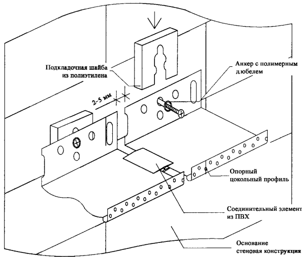
Рисунок 1 – Схема монтажа опорного (цокольного) профиля
