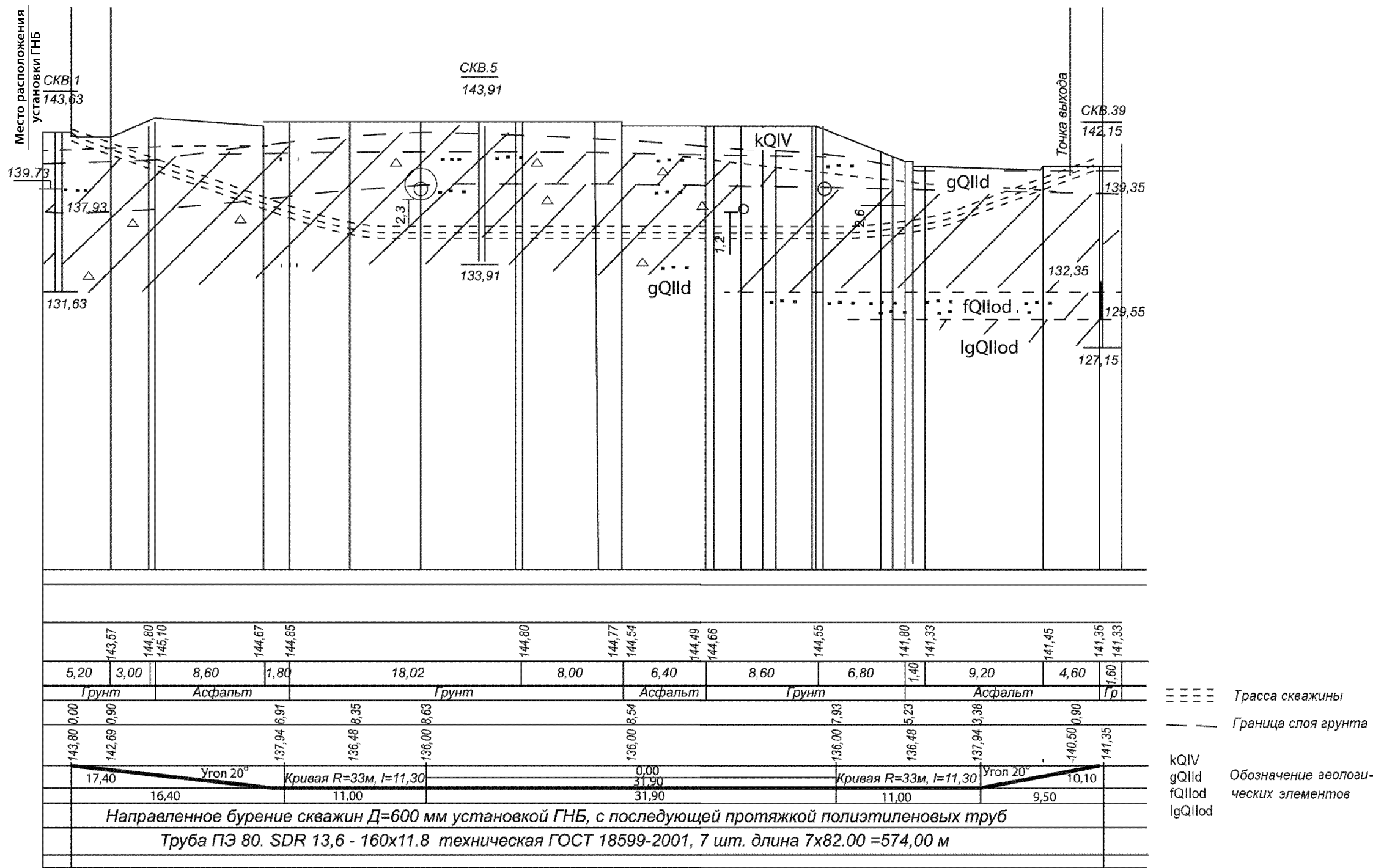
7.1 – Пример построения продольного профиля трассы скважины ГНБ
