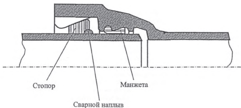
Рисунок 7.3 – Разрез раструбно-замкового соединения
