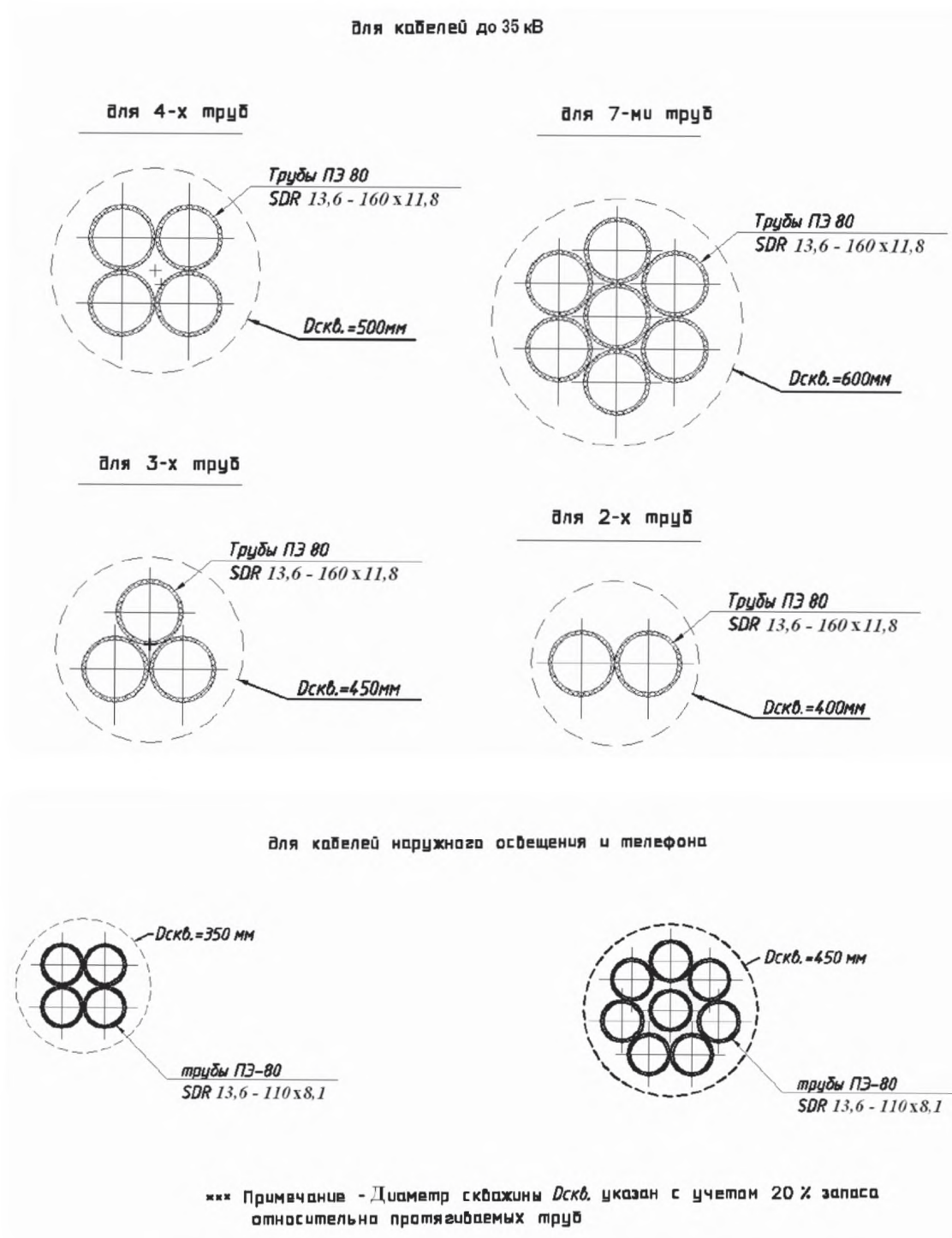
Рисунок 7.4 – Сечения закрытых переходов для прокладки кабелей
