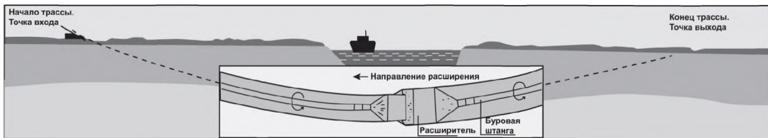
Рисунок 8.4 – Расширение скважины
