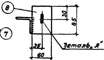
МД4-8 обратно чертежу
